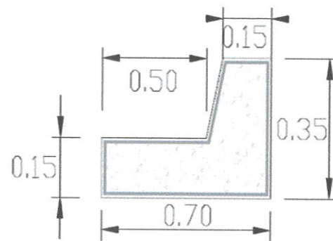
DETALLE DE GUARNICION TIPO "L" (SIN ESCALA)
