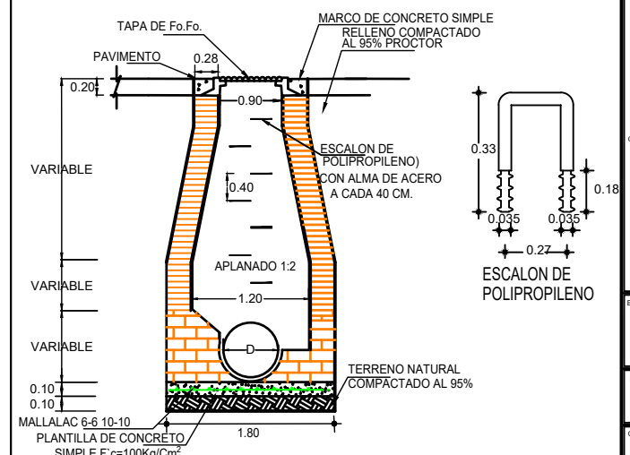
CORTE A-A POZO DE VISITA COMÚN
