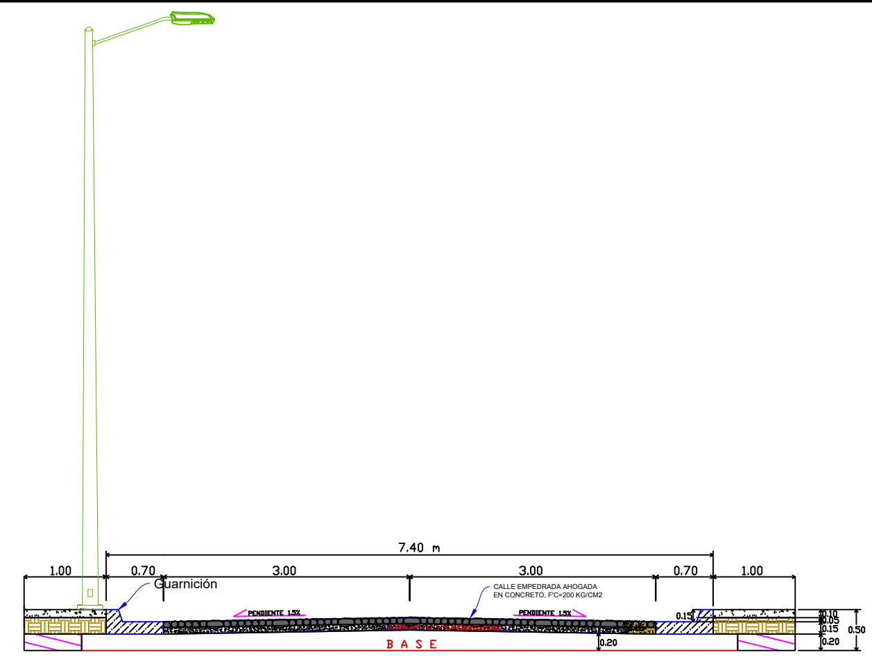
SECCION TRANSVERSAL (PIEDRA AHOGADA EN CONCRETO) LONG: 25.00 MTRS
