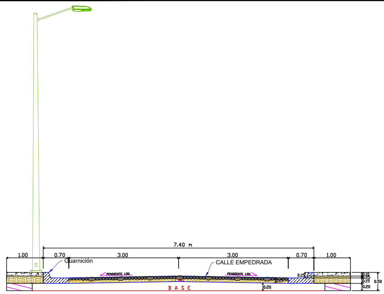
SECCION TRANSVERSAL TIPO
