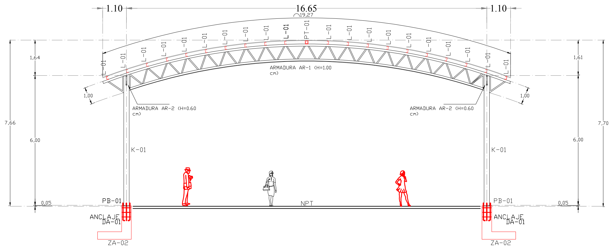
CORTE TRANSVERSAL
