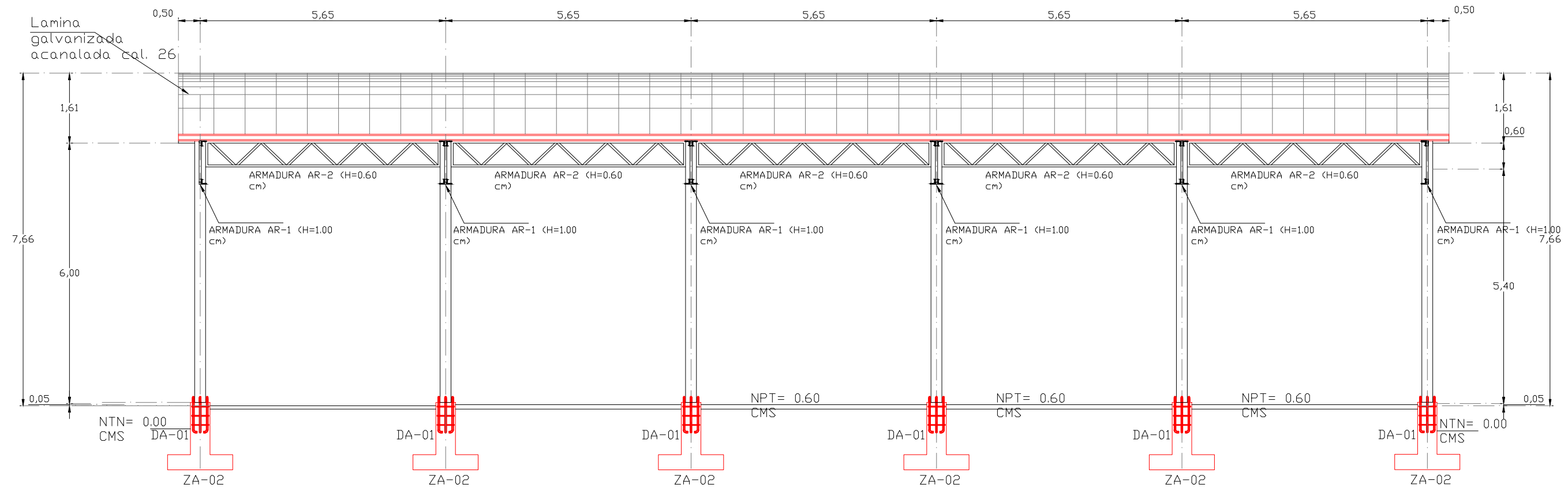
CORTE LONGITUDINAL
