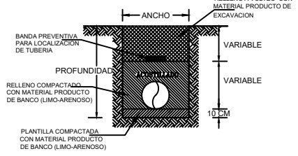
SECCION DE EXCAVACION
