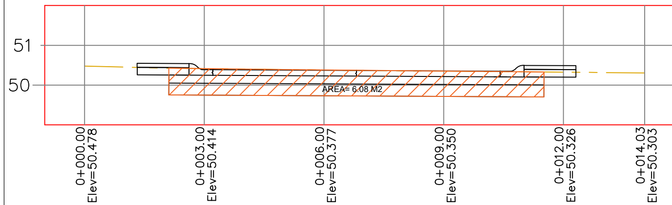
PERFIL 0+141.10
