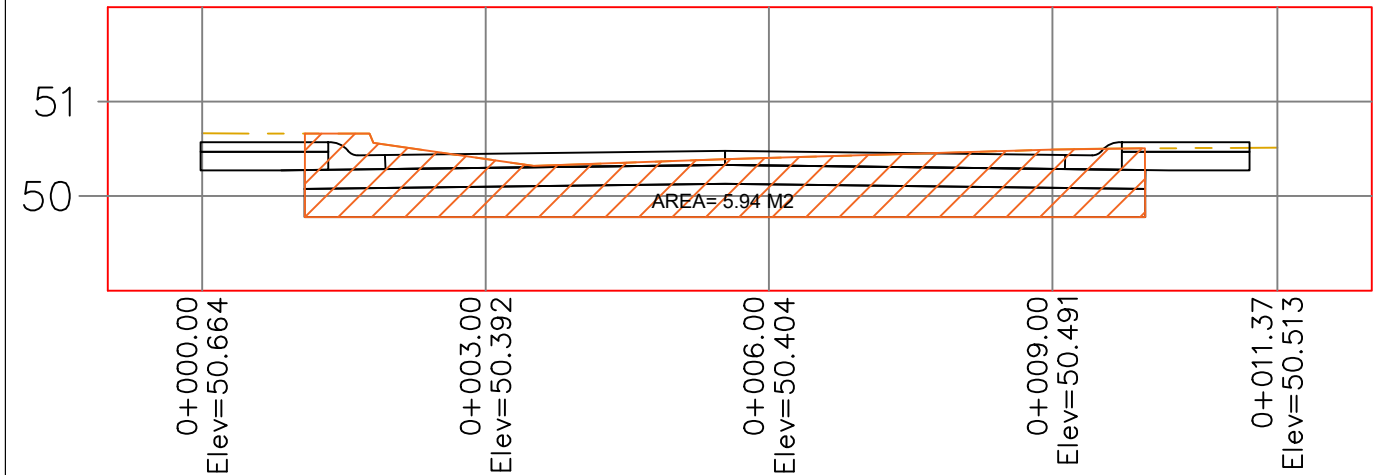
PERFIL 0+100
