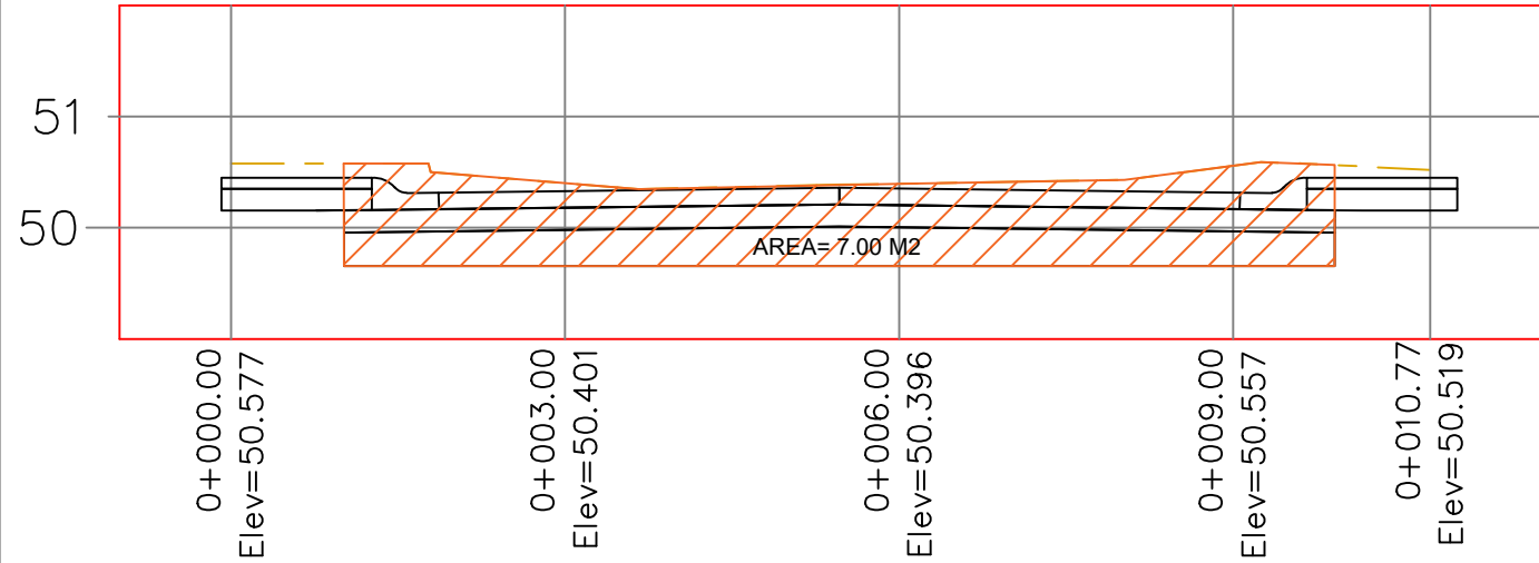
PERFIL 0+080
