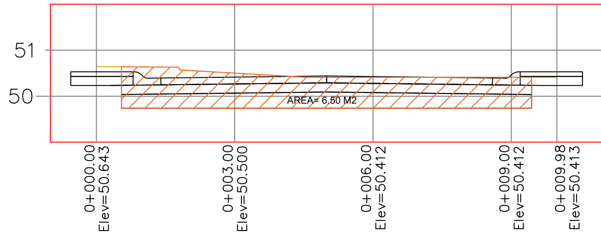
PERFIL 0+120
