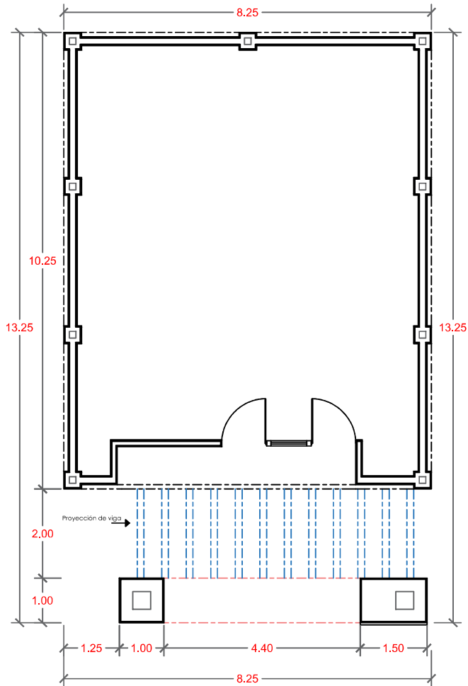
PLANTA ARQUITECTÓNICA
