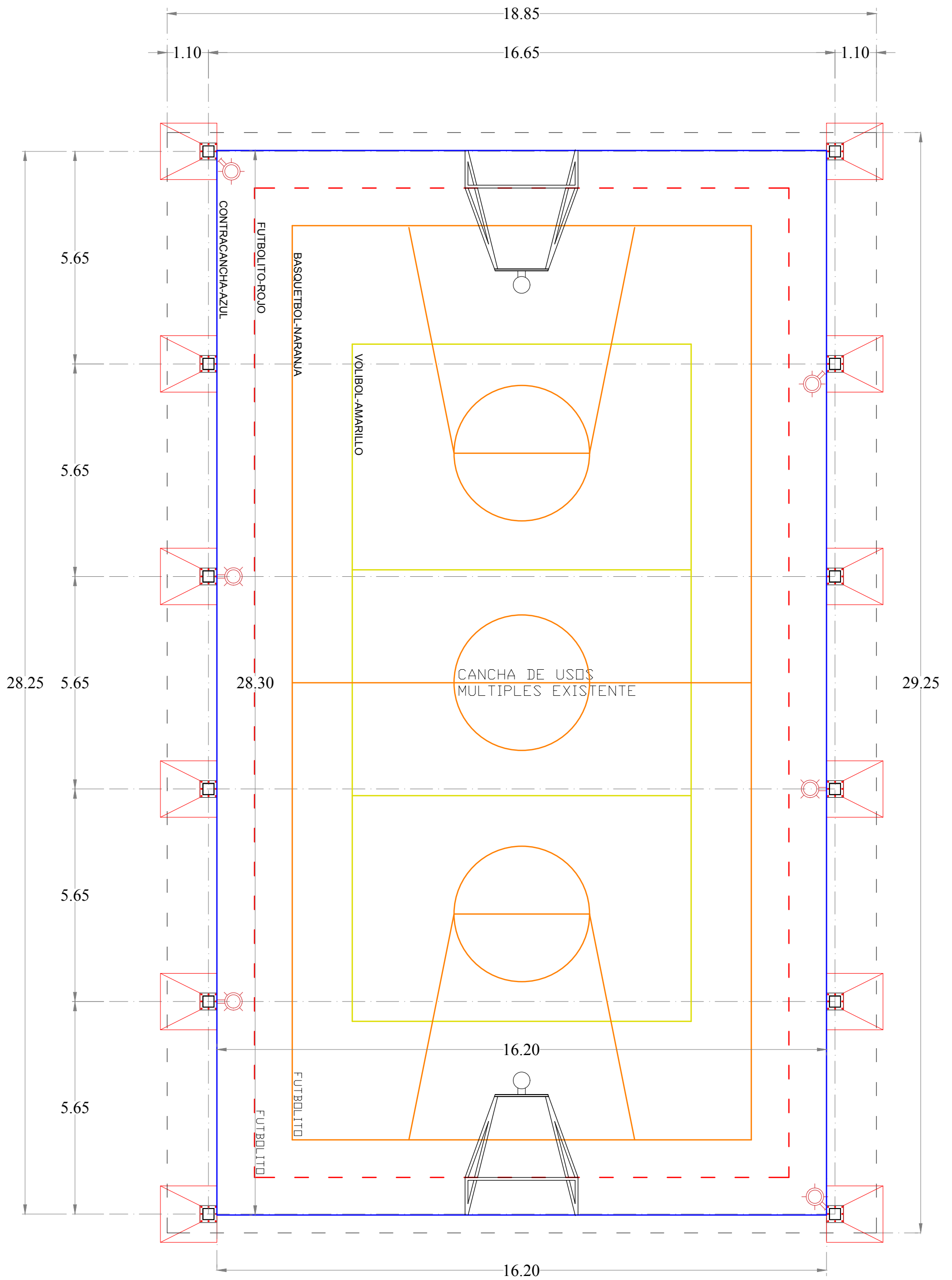
PLANTA DE CIMENTACION
