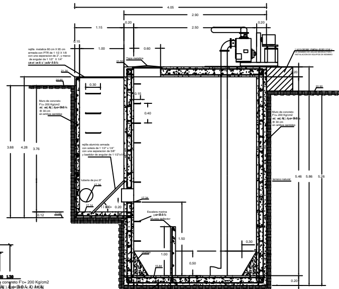
CORTE X-X'
