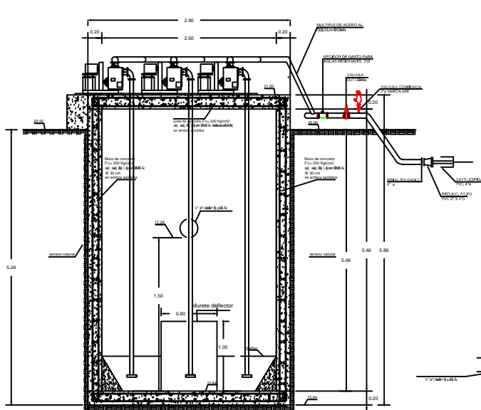
CORTE Y-Y'
