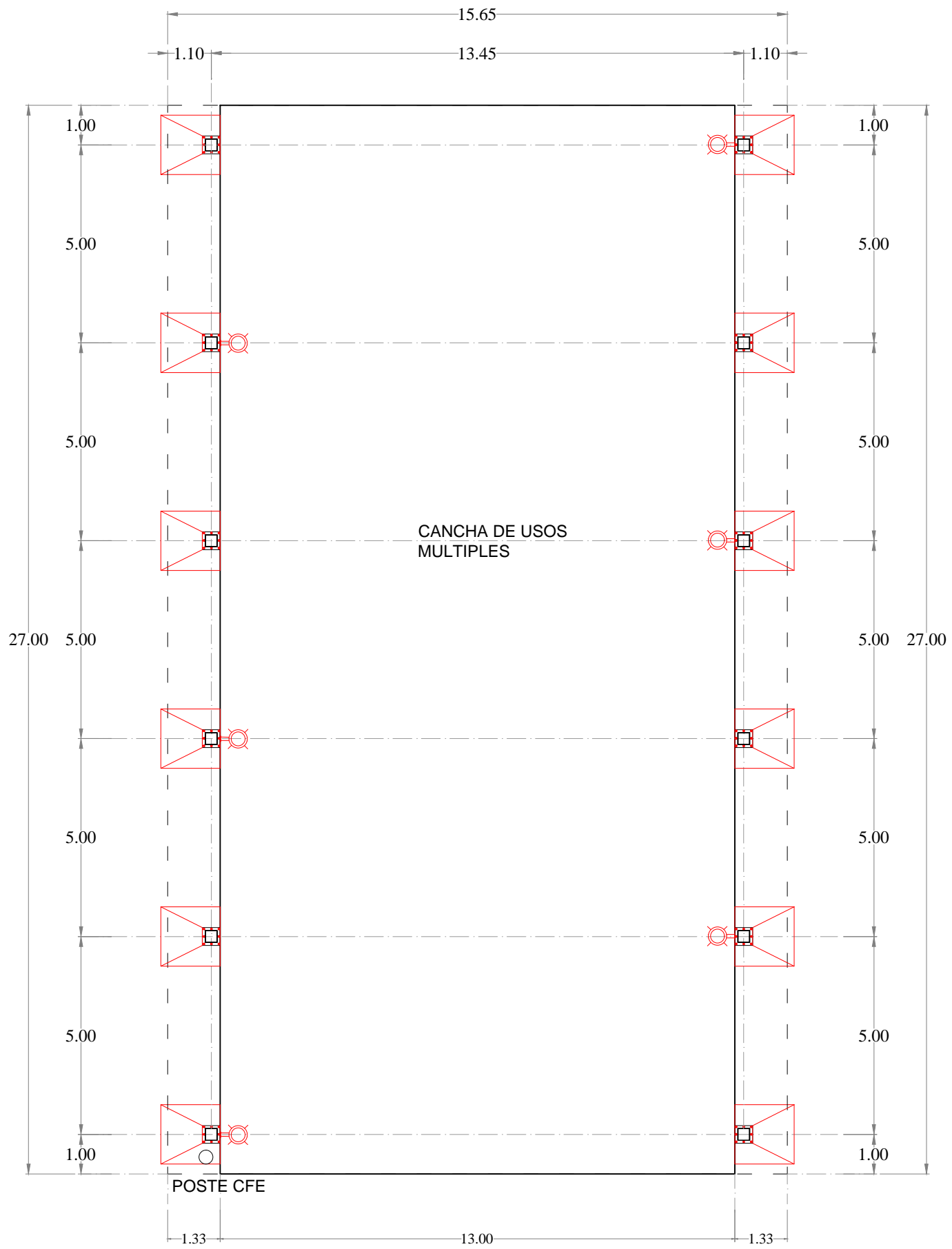
PLANTA DE CIMENTACION
