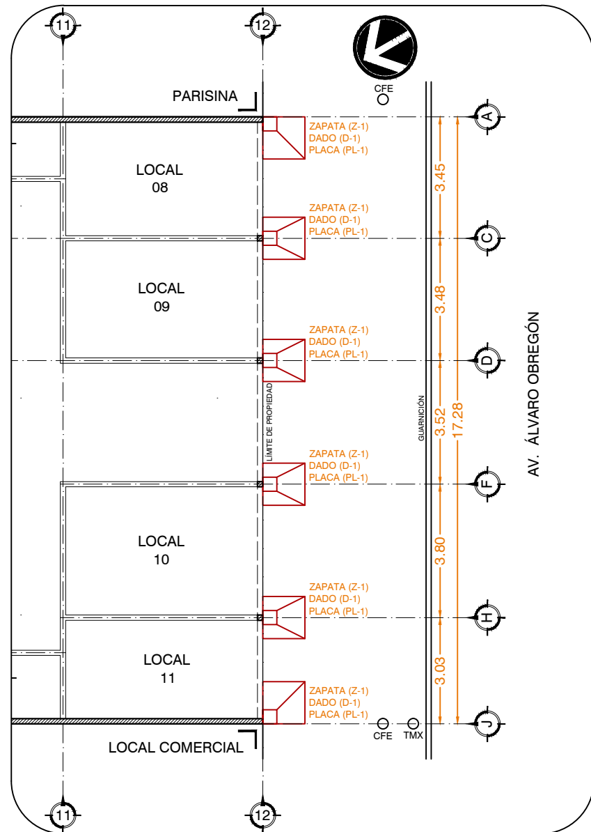
PLANTA DE CIMENTACION ESC. 1:150
