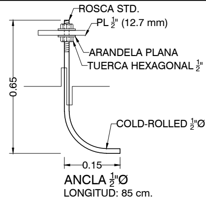
DETALLES DE ANCLAJE EN CIMENTACION ESC. 1:10
