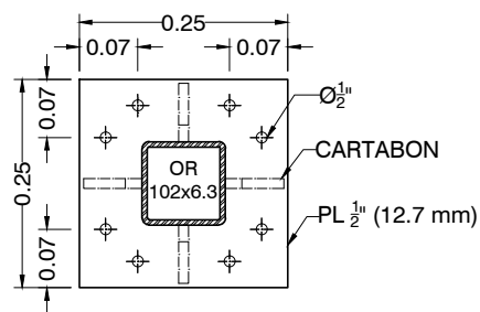
PLACA BASE (PL-1) DIMENSIONES: 25 x 25 cm. ESPESOR: 1/2" (12.7 mm)
