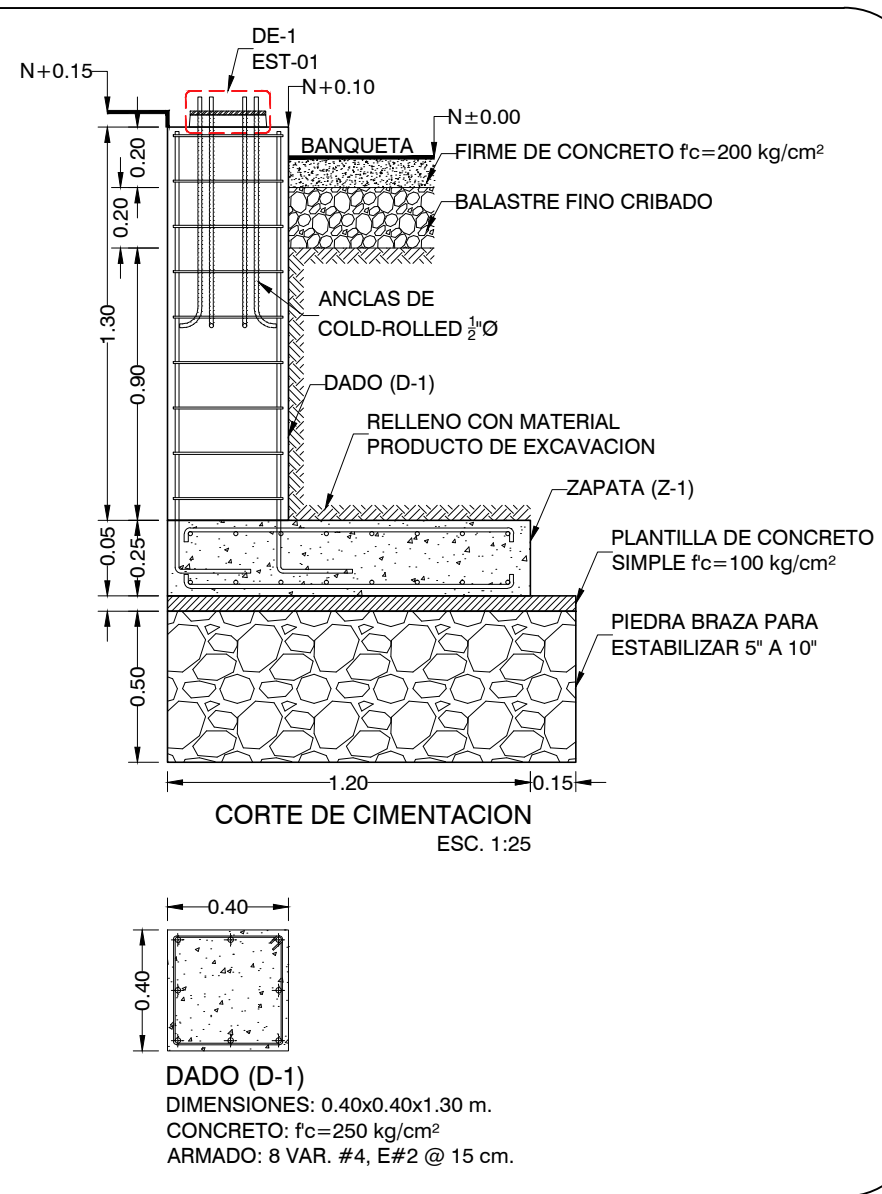
DETALLES DE CIMENTACION ESC. 1:25
