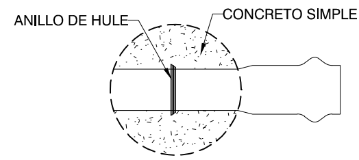
UNION DE TUBO PVC EN POZO DE VISITA ESC. 1:25
