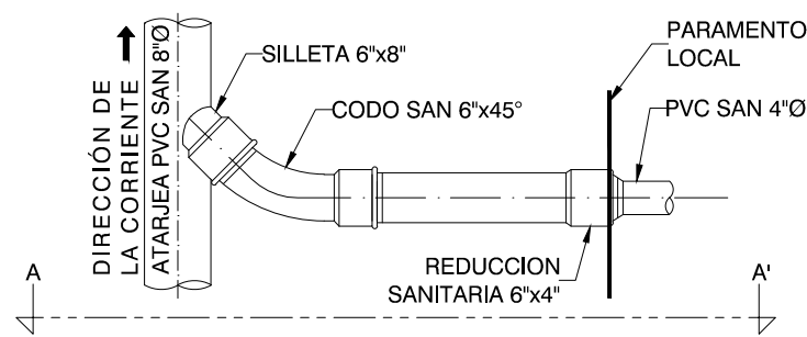
DESCARGA DE LOCALES (VISTA B-B') ESC. 1:25
