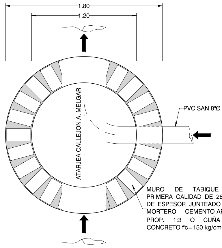
PLANTA POZO DE VISITA ESC. 1:25
