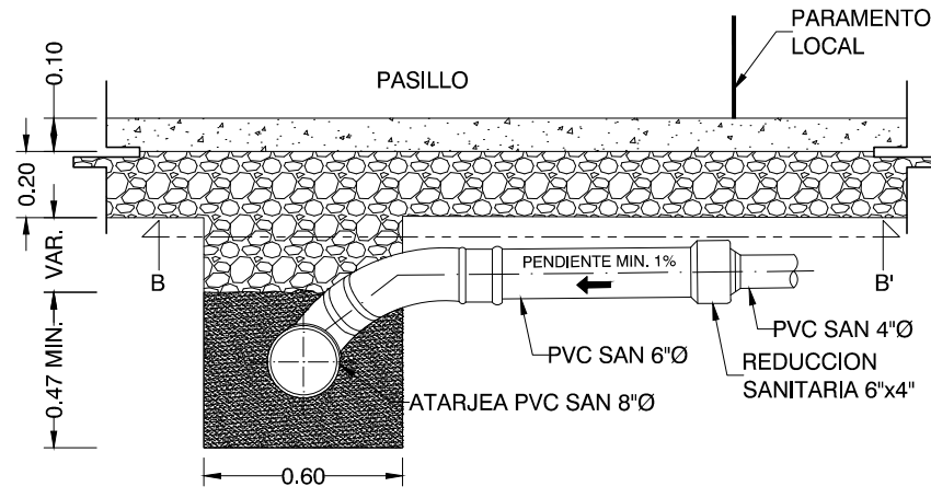
DESCARGA DE LOCALES (VISTA A-A') ESC. 1:25
