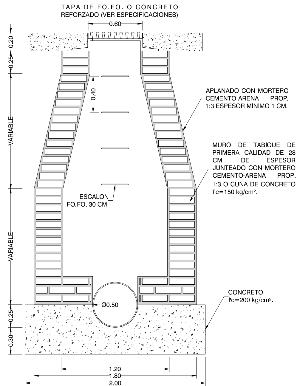
ELEVACION POZO DE VISITA PARA PROFUNDIDADES MAYORES A 2.50 M. ESC. 1:25
