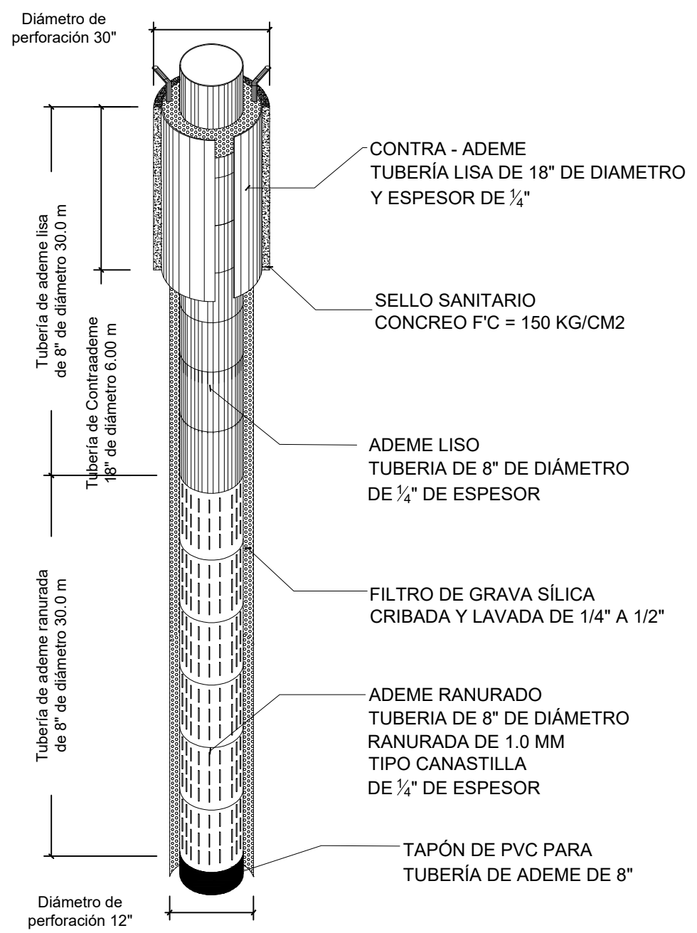
DISEÑO DE POZO PROFUNDO
