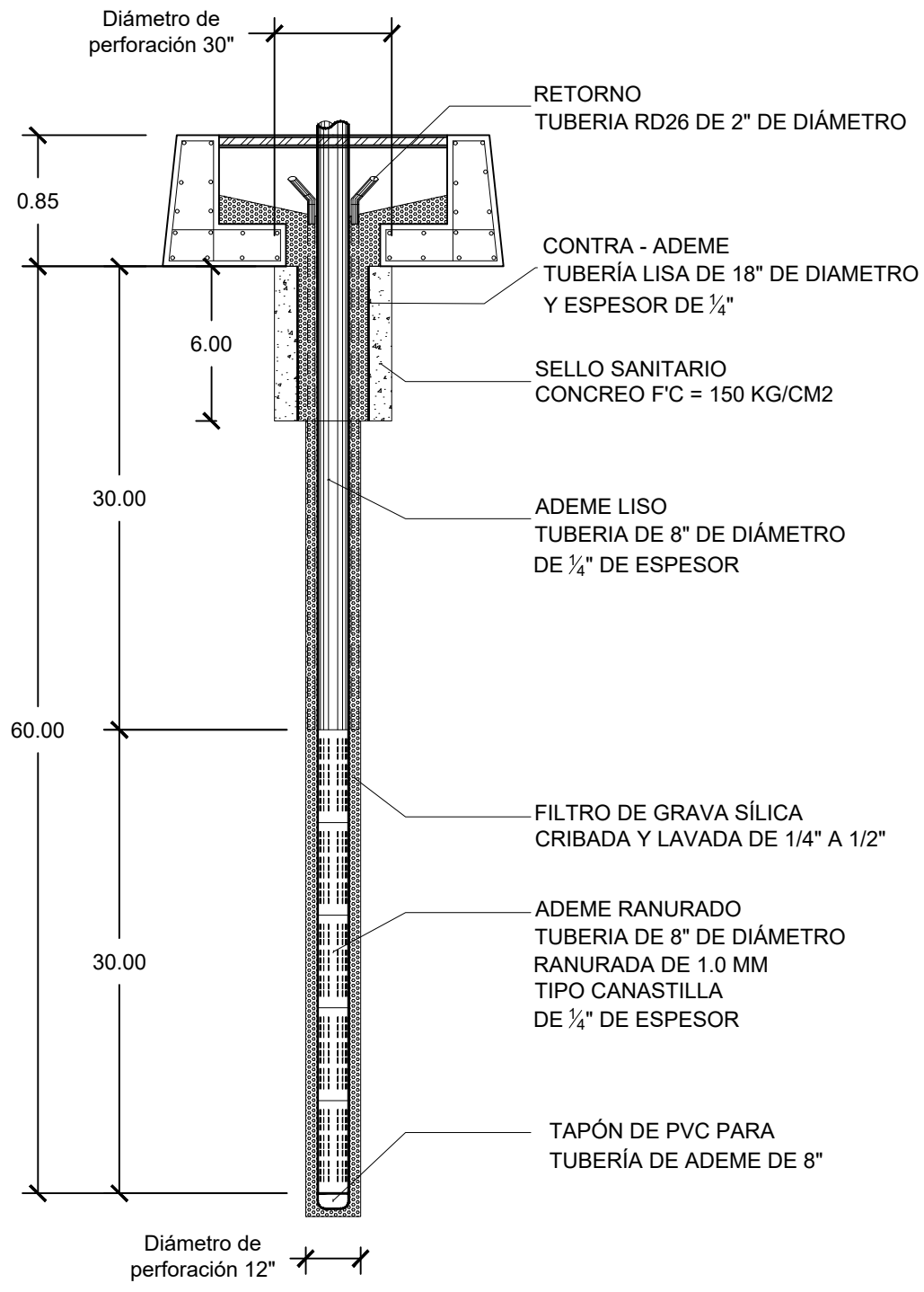
CORTE DE POZO PROFUNDO
