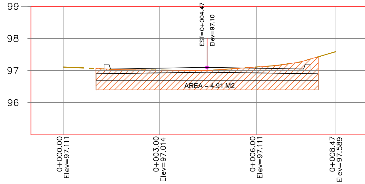
PERFIL 0+180
