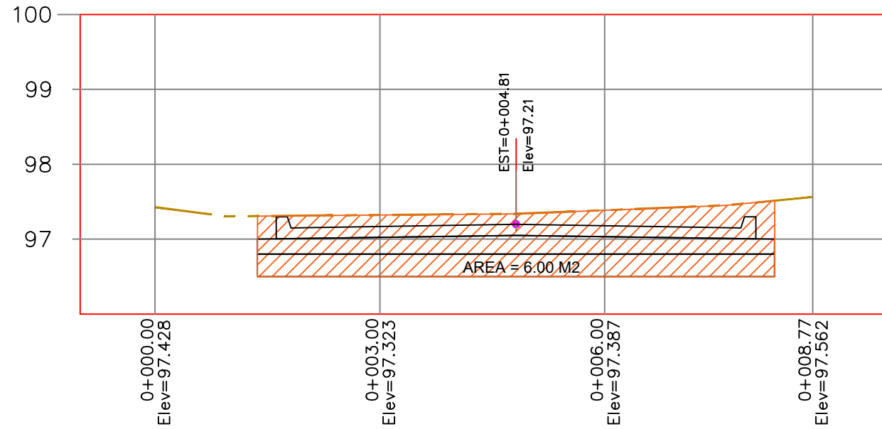
PERFIL 0+160
