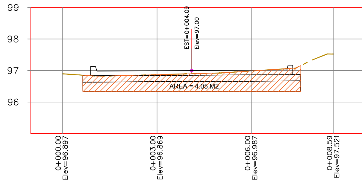
PERFIL 0+191.8
