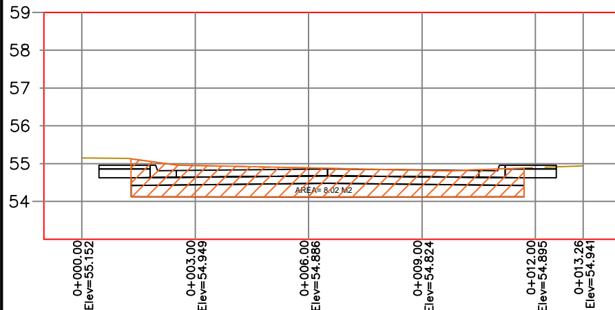
PERFIL 3
