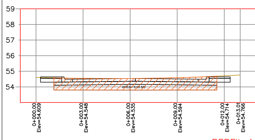
PERFIL 1
