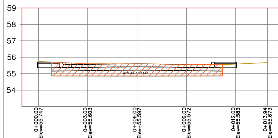
PERFIL 8
