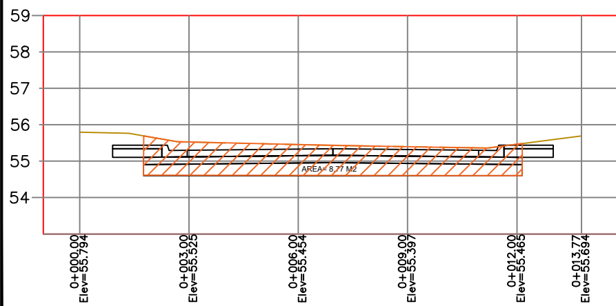
PERFIL 6
