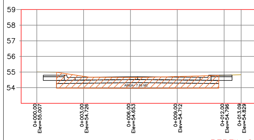
PERFIL 2
