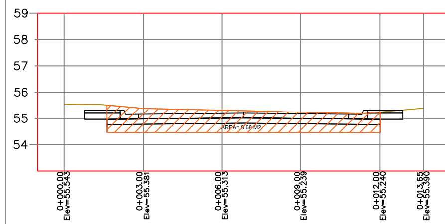
PERFIL 5
