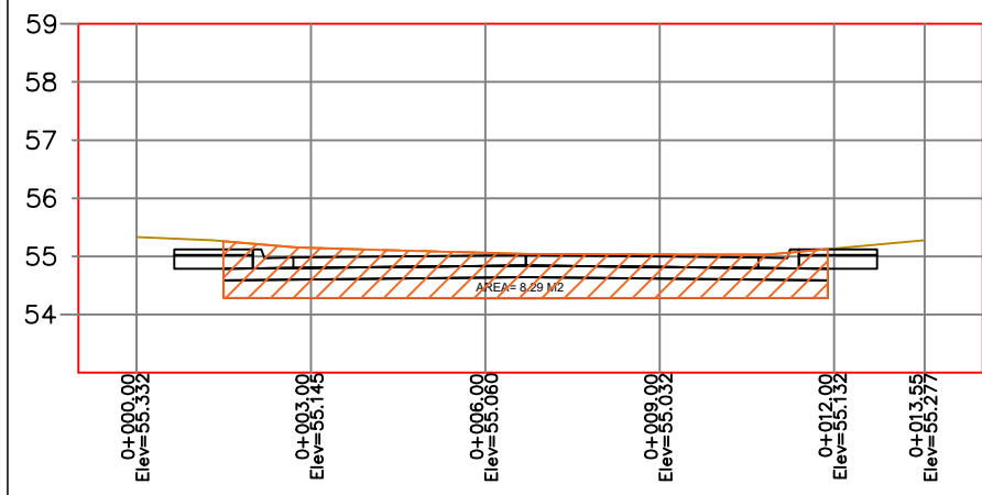
PERFIL 4
