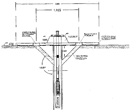
BASE PARA EQUIPO DE BOMBEO CORTE A-A'
