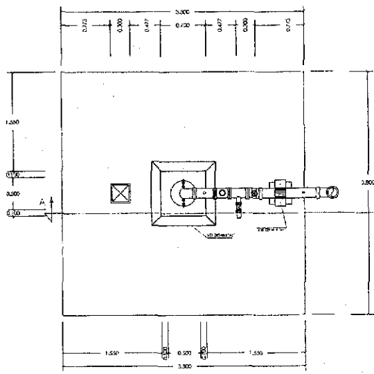
PLANTA CON ARREGLOS HIDRAULICOS ESC. 1:25.
