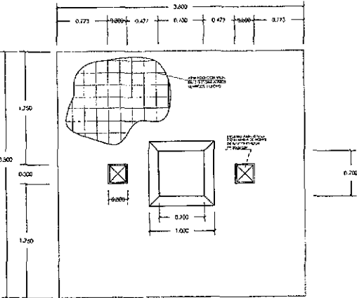
PLANTA CON BASE PARA ARREGLOS HIDRAULICOS. ESC. 1:25.
