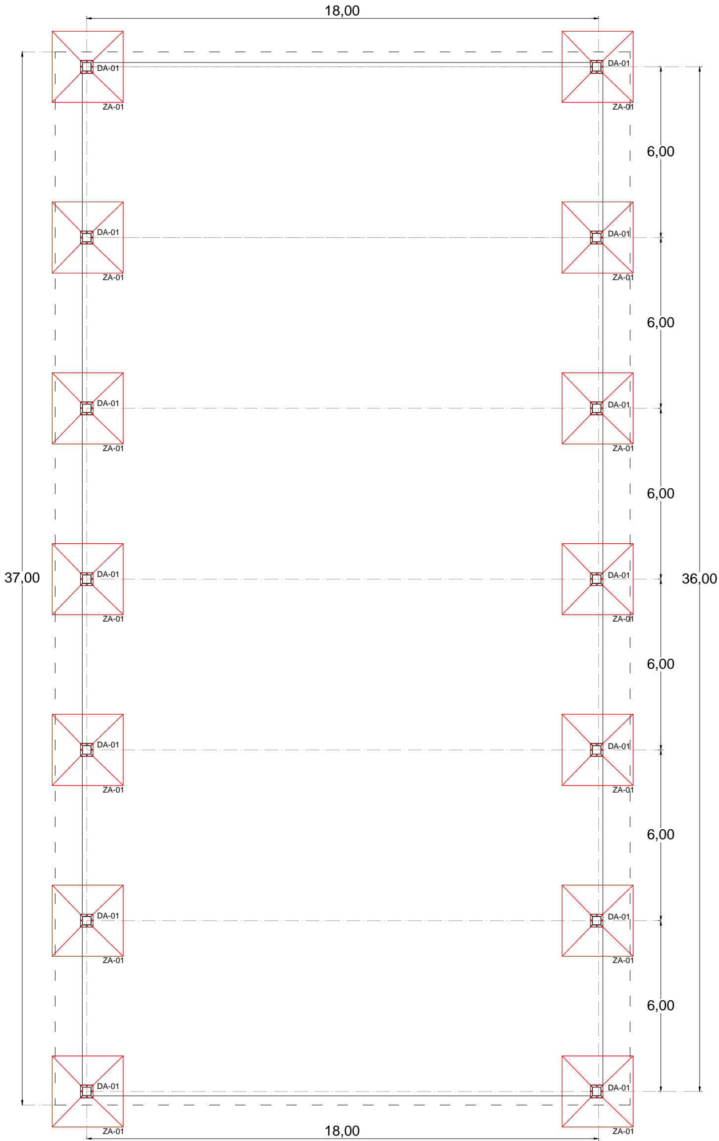
PLANTA DE CIMENTACION
