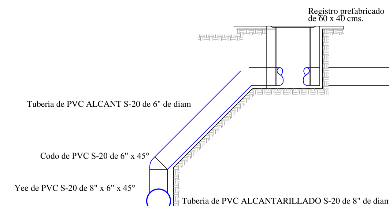
DETALLE DE CONEXION.- Descarga domiciliaria.-
