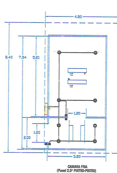
TRAZO PLANTA OPCION I CAMARA FRIA INSTALACION MECANICA-INSTALACION ELECTRICA INSTALACION ELECTRICA DE ILUMINACION
