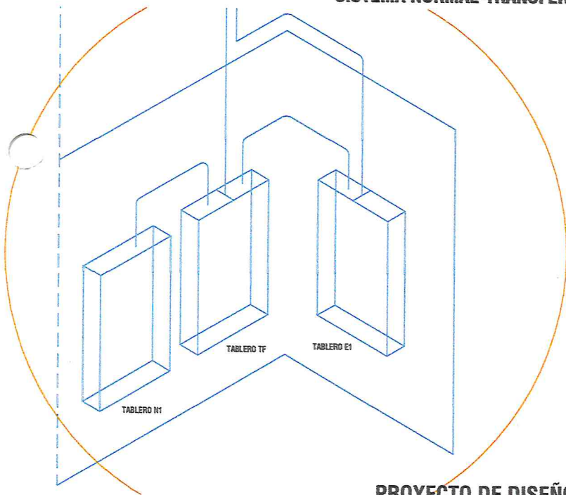
TRAZO ISOMETRICO OPCION I CAMARA FRIA INSTALACION ELECTRICA DE EMERGENCIA SISTEMA NORMAL-TRANSFERENCIA-SISTEMA EMERGENCIA
