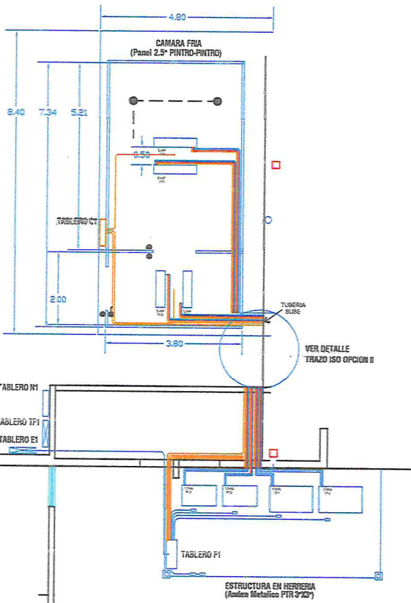
TRAZO PLANTA OPCION II CAMARA FRIA INSTALACION MECANICA-INSTALACION ELECTRICA INSTALACION ELECTRICA DE CONTROL
