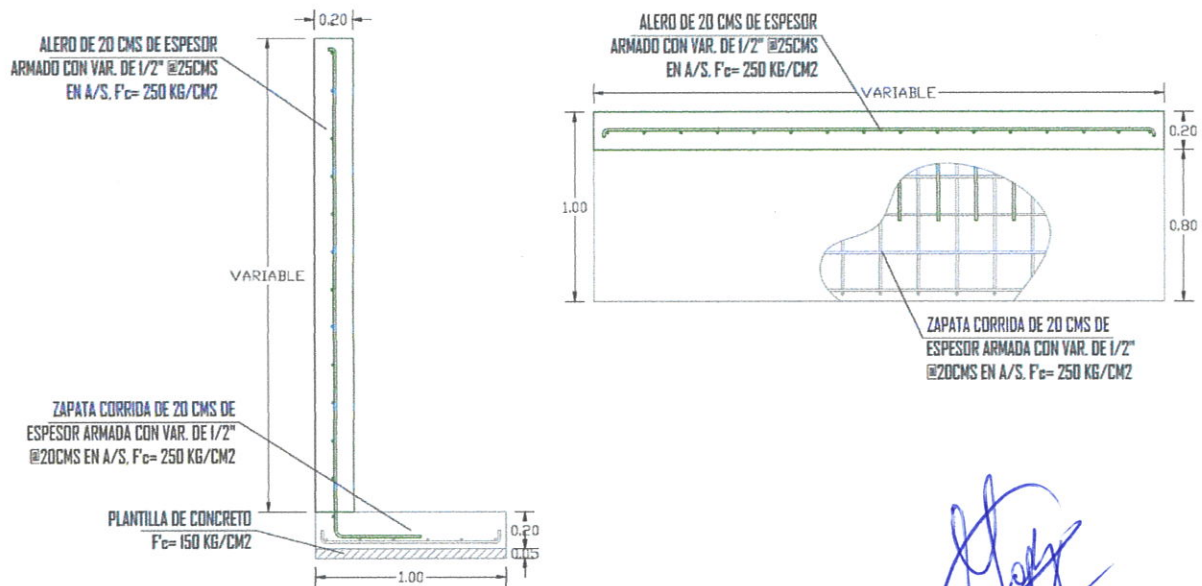
DETALLES DE ALERO
