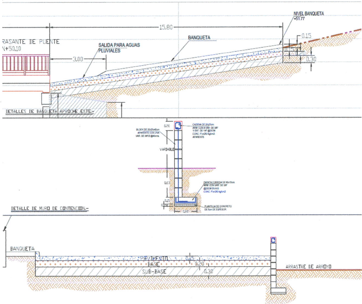
DETALLES DE BANQUETA
