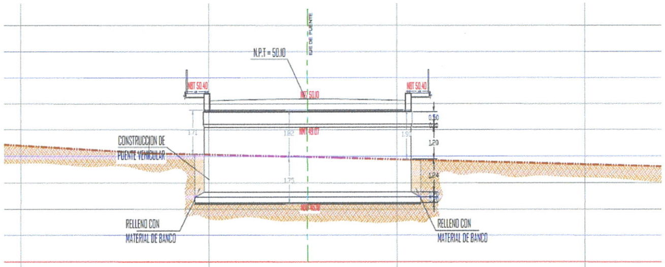
PERFIL CENTRO DE ARROYO
