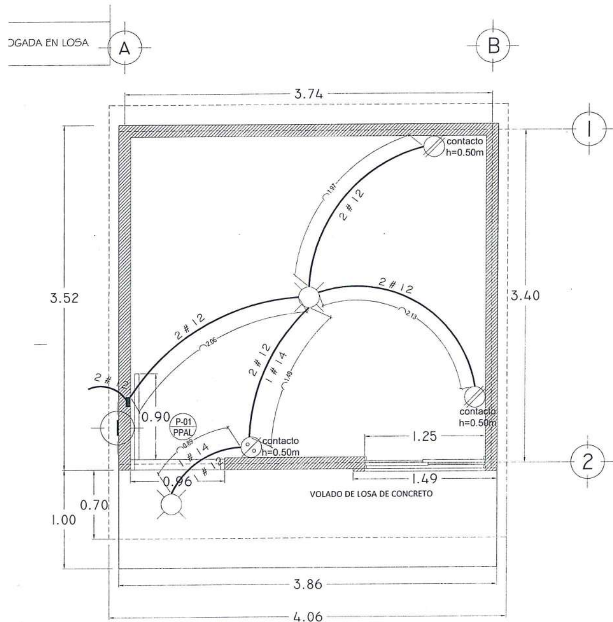
PLANTA DE INSTALACIÓN ELÉCTRICA
