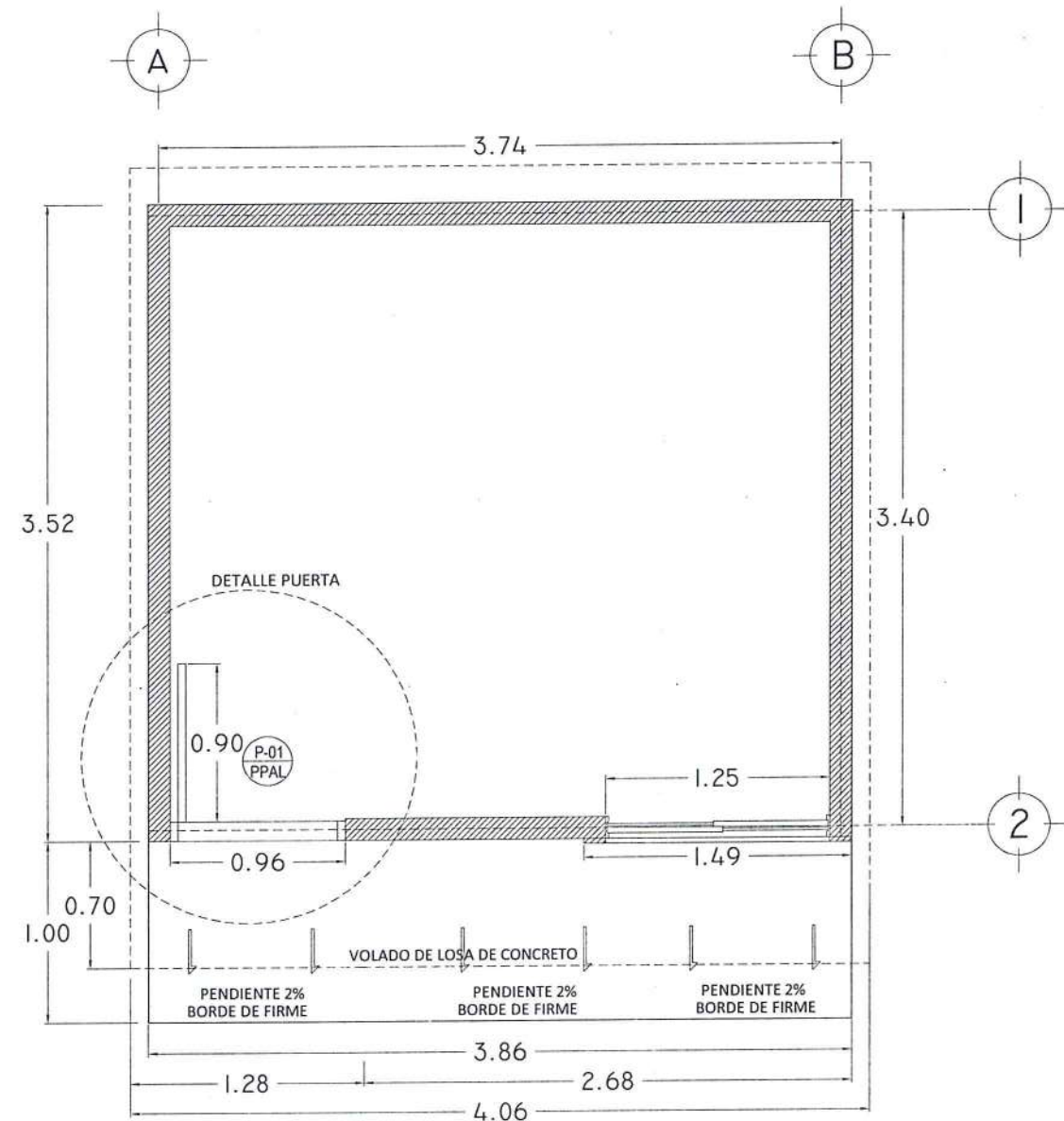
PLANTA ARQUITECTÓNICA
