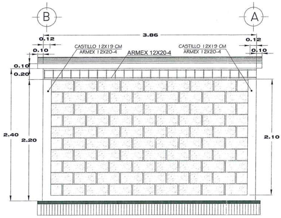
ALZADO POSTERIOR
