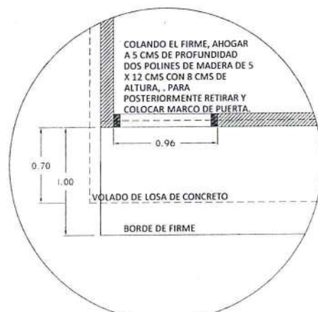
PLANTA DETALLE DE PREPARACION PARA ANCLAJE DE PUERTA
