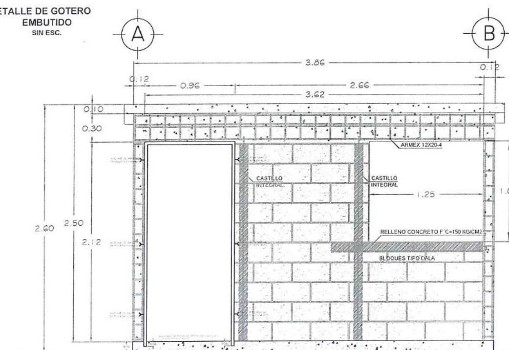
ALZADO FRONTAL ESTRUCTURAL
