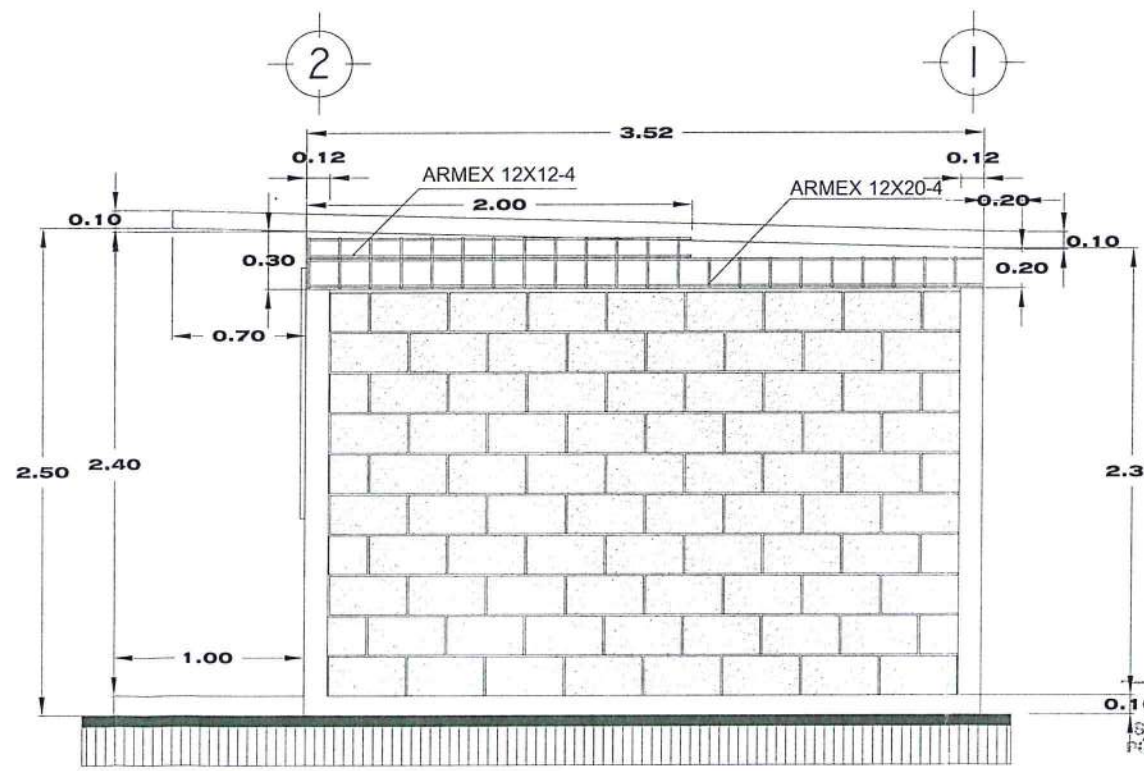
ALZADO LATERAL
