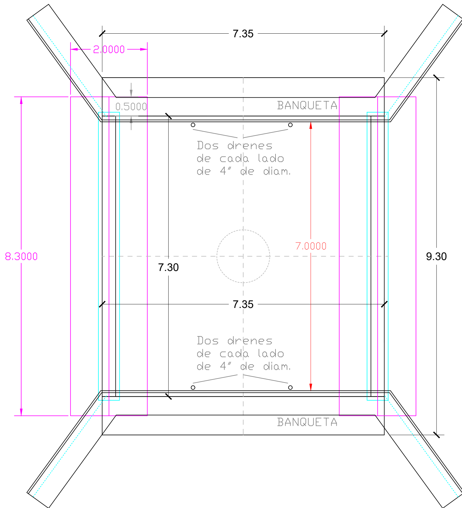
-DETALLES DE PUENTE VEHICULAR.- ESCALA= 1:60
