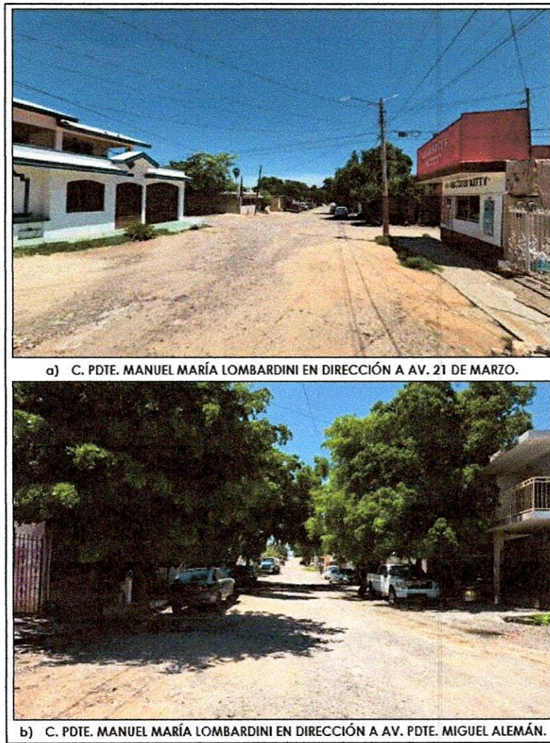
Figura 1: Visita al sitio de la obra en la calle Pdte. Manuel maría Lombardini, tramo entre av. Pdte. Miguel Alemán y av. 21 de Marzo, colonia Lázaro Cárdenas, ciudad de Culiacán Rosales, municipio de Culiacán, Sinaloa.
