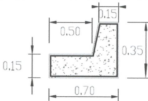
DETALLE DE GUARNICION TIPO "L" (SIN ESCALA)
