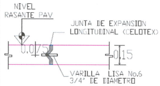
DETALLE DE JUNTA CONSTRUCTIVA
