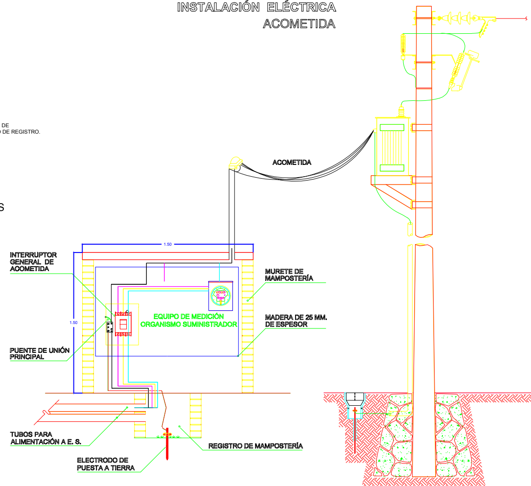
ACOMETIDA ELÉCTRICA
