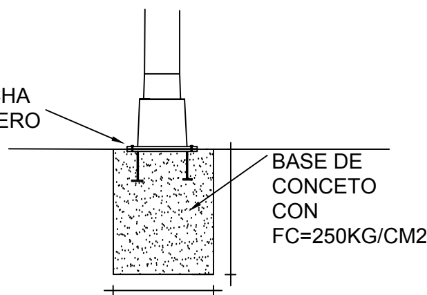
DETALLE DE ARBORTANTE METALICO S/E.
