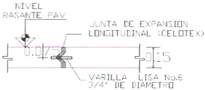
DETALLE DE JUNTA CONSTRUCTIVA
