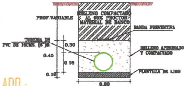
EN TIERRA SECCION DE DESCARGA 15 CMS.
