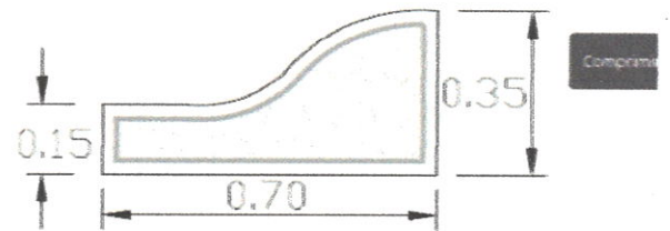
DETALLE DE GUARNICION TIPO "PECHO PALOMA"
