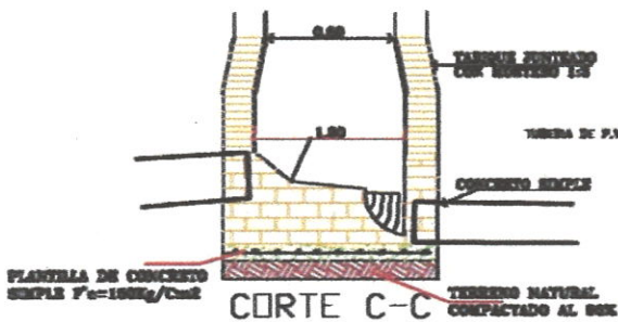
DETALLES DE POZO DE VISITA "COMUN" CON TUBERIA DE P.V.C.
