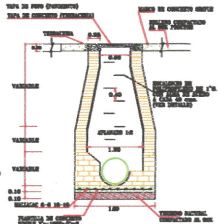
POZO DE VISITA COMUN
