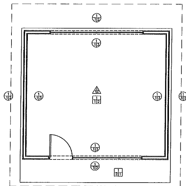
4 ACABADOS EN PLANTA ARQUITECTÓNICA
