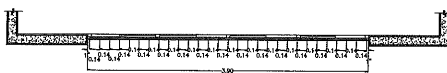
3 HERRERIA EN FACHADA POSTERIOR – TALLERES Y LABORATORIOS ESC. 1:50
