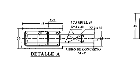
DETALLE DE MUROS
