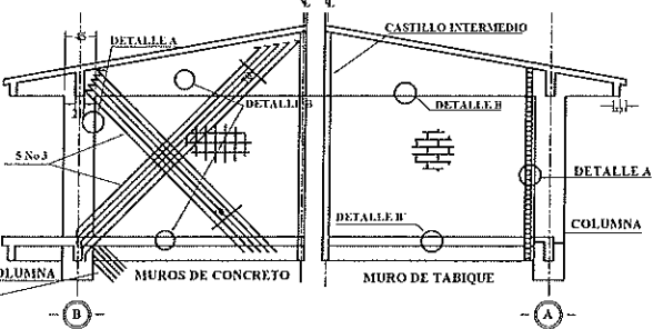
CORTE J-J
