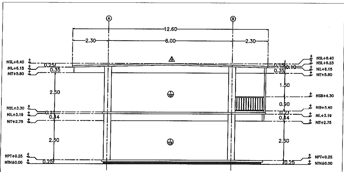
FACHADA LATERAL
