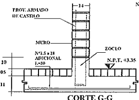
CORTE G-G
