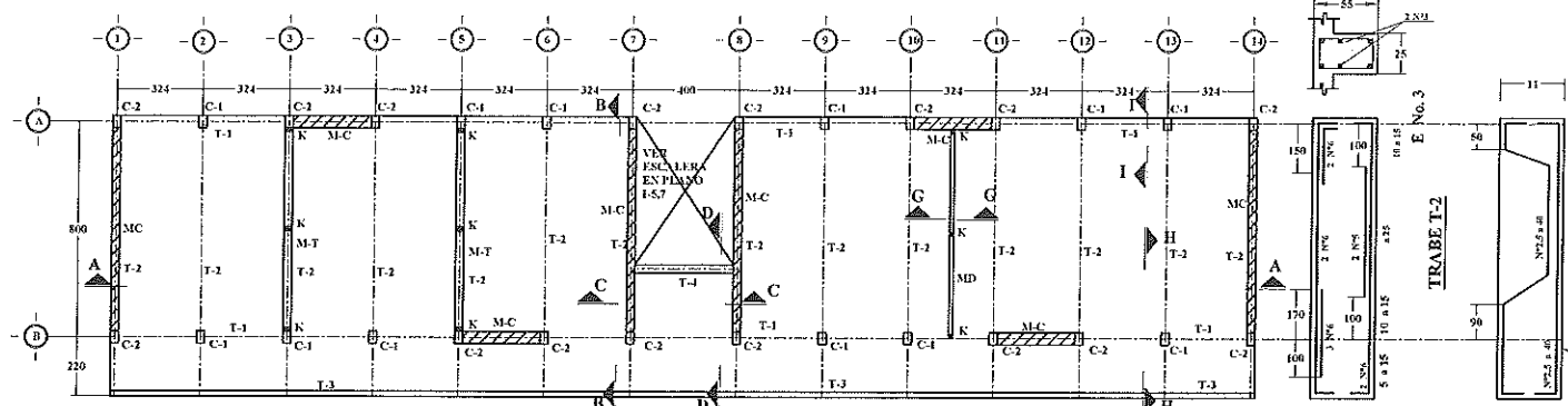
PLANTA DE ENTREPISO
