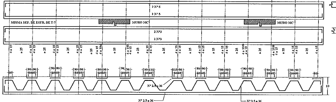
CORTE F-F
