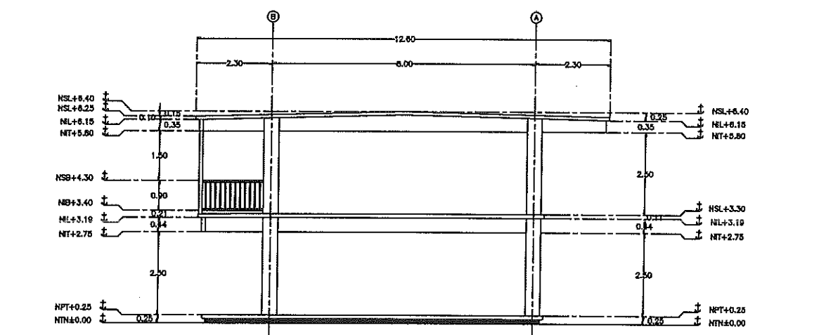
4 FACHADA LATERAL ESC. 1:75
