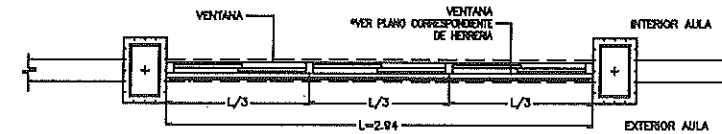
2 CANCELERIA EN FACHADA POSTERIOR - MUROS BAJOS
