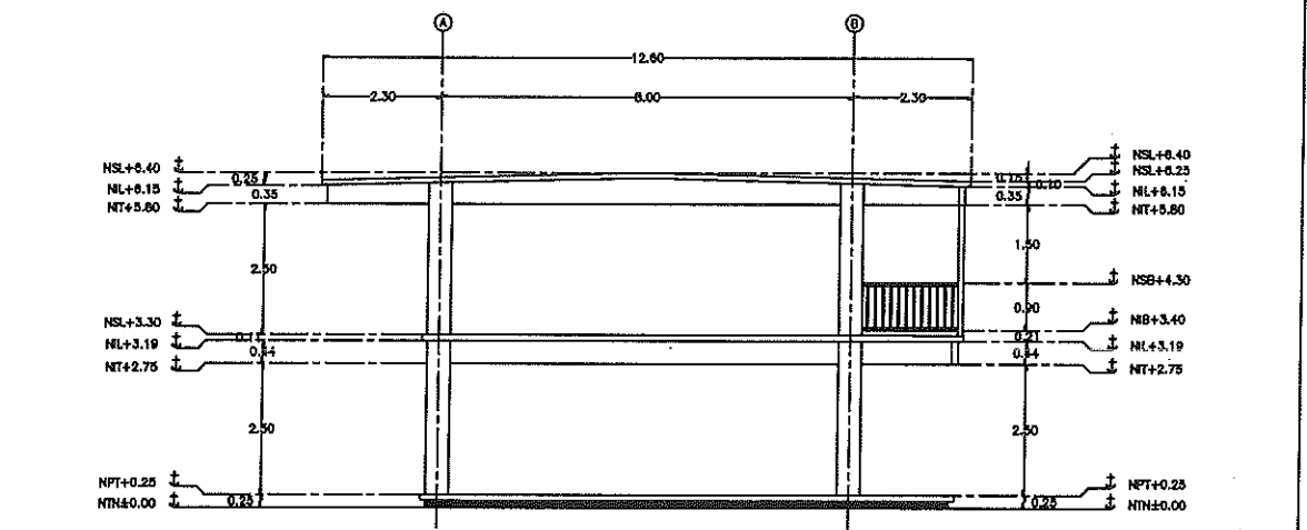
3 FACHADA LATERAL ESC. 1:75
