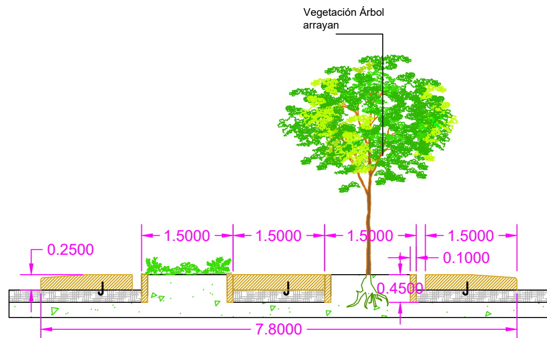
SECCIÓN A
