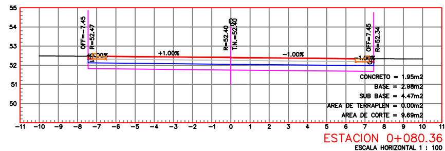
ESTACION 0+080.36 ESCALA HORIZONTAL 1 : 100 ESCALA VERTICAL 1 : 100
