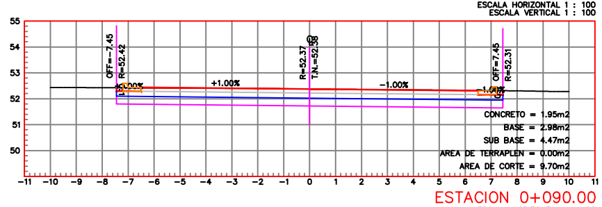
ESTACION 0+090.00 ESCALA HORIZONTAL 1 : 100 ESCALA VERTICAL 1 : 100
