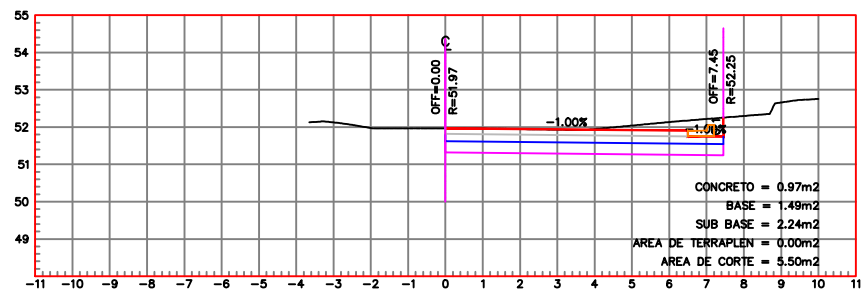
ESTACION 0+128.49 ESCALA HORIZONTAL 1 : 100 ESCALA VERTICAL 1 : 100
