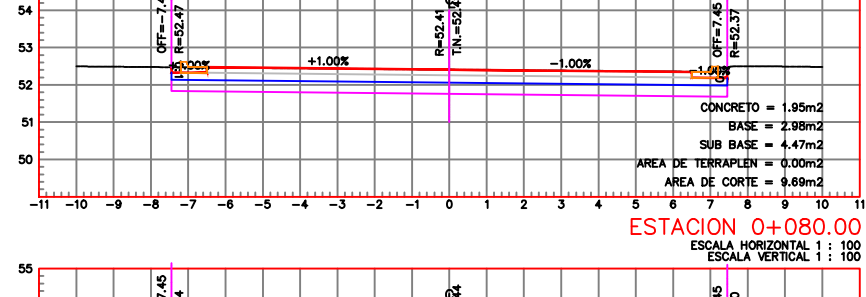
ESTACION 0+080.00 ESCALA HORIZONTAL 1 : 100 ESCALA VERTICAL 1 : 100
