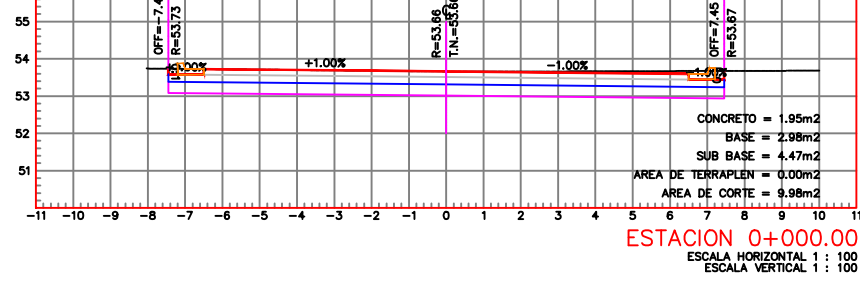
ESTACION 0+000.00 ESCALA HORIZONTAL 1 : 100 ESCALA VERTICAL 1 : 100
