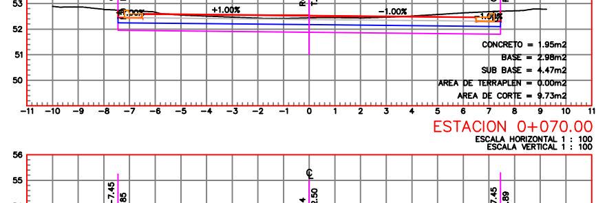
ESTACION 0+070.00 ESCALA HORIZONTAL 1 : 100 ESCALA VERTICAL 1 : 100
