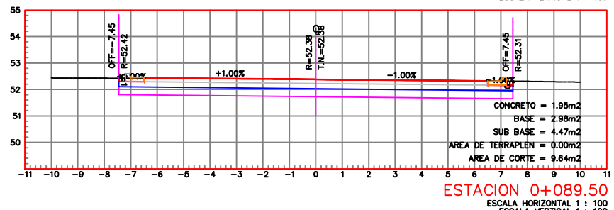
ESTACION 0+089.50 ESCALA HORIZONTAL 1 : 100 ESCALA VERTICAL 1 : 100
