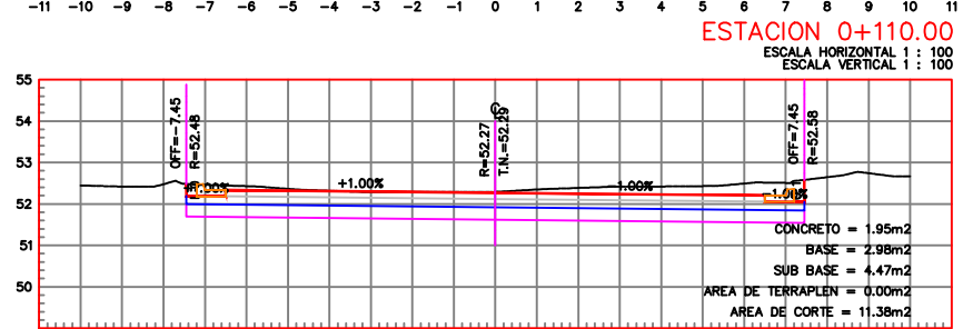
ESTACION 0+100.00 ESCALA HORIZONTAL 1 : 100 ESCALA VERTICAL 1 : 100
