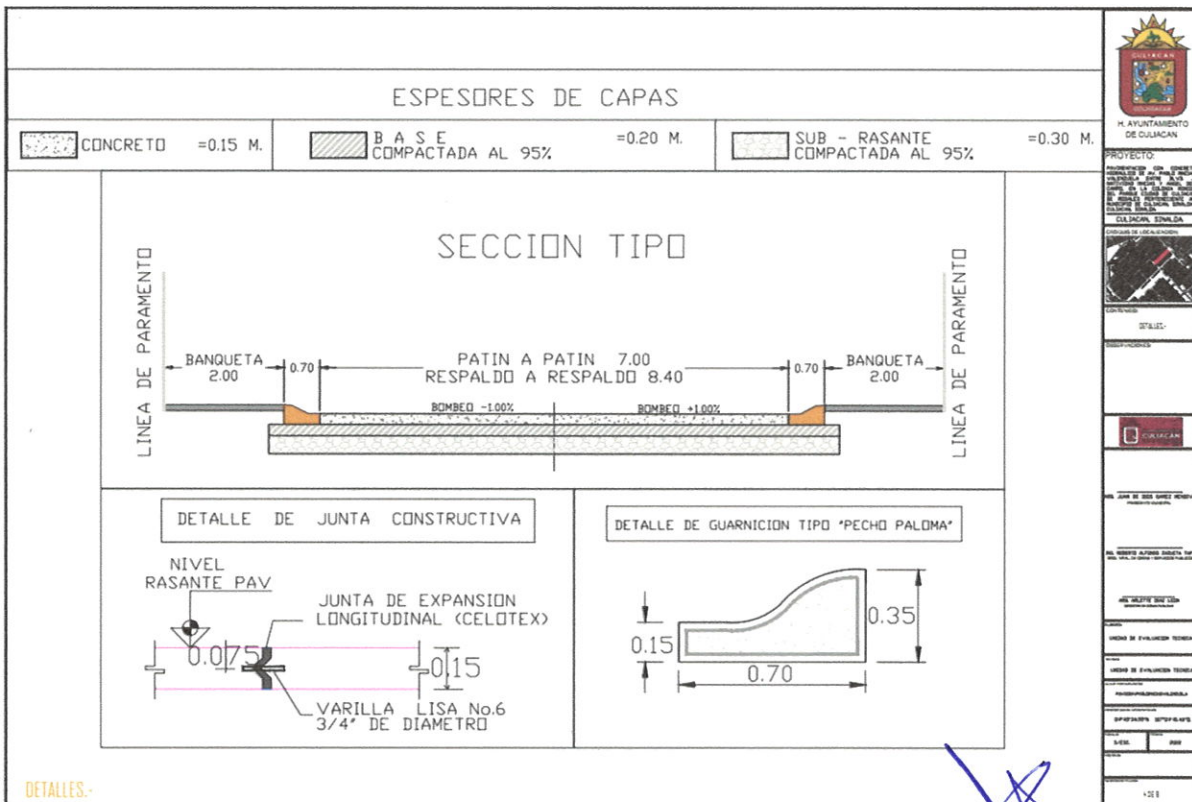
Plano de Detalles de Pavimento
