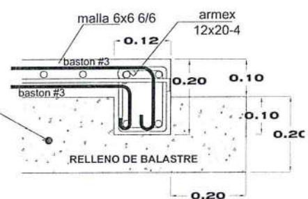
DETALLE DE CIMENTACION CORTE A-A'
