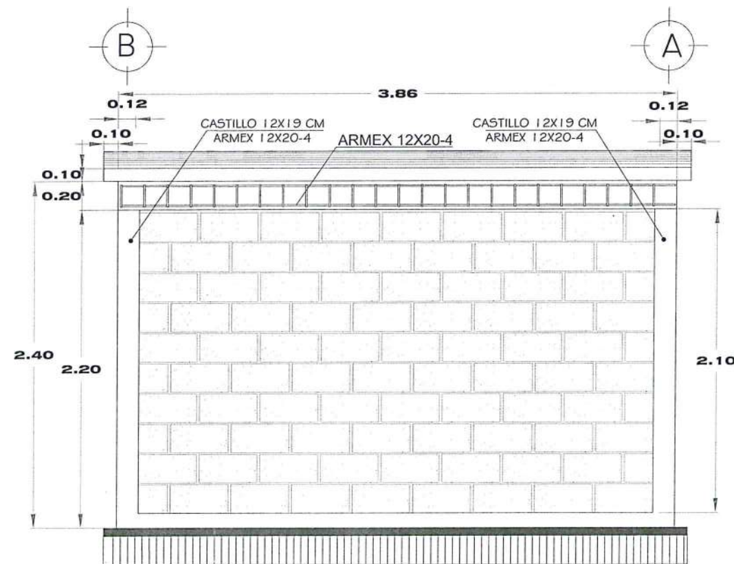
ALZADO POSTERIOR
