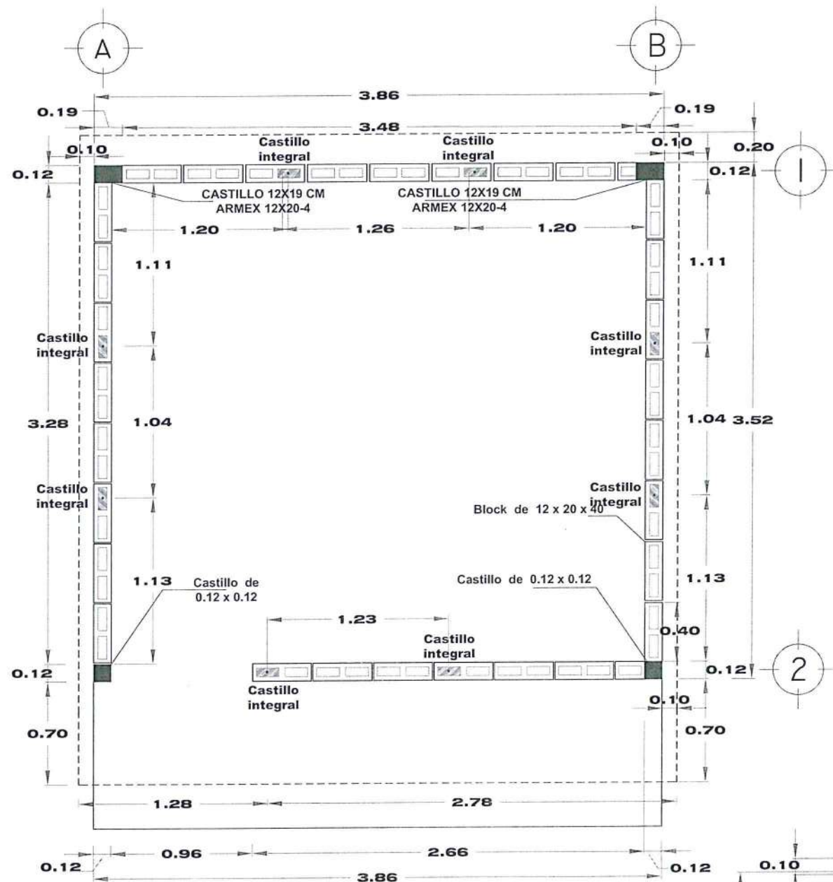
PLANTA DE MODULACIÓN DE BLOQUES EN MUROS
