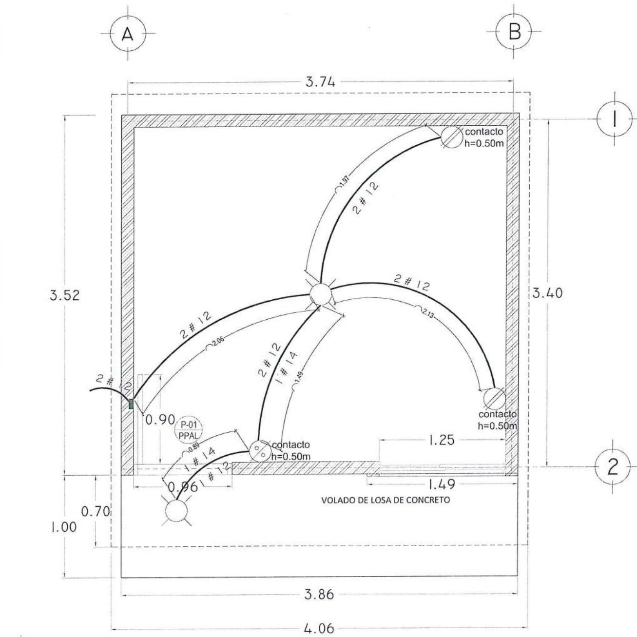
PLANTA DE INSTALACIÓN ELÉCTRICA
