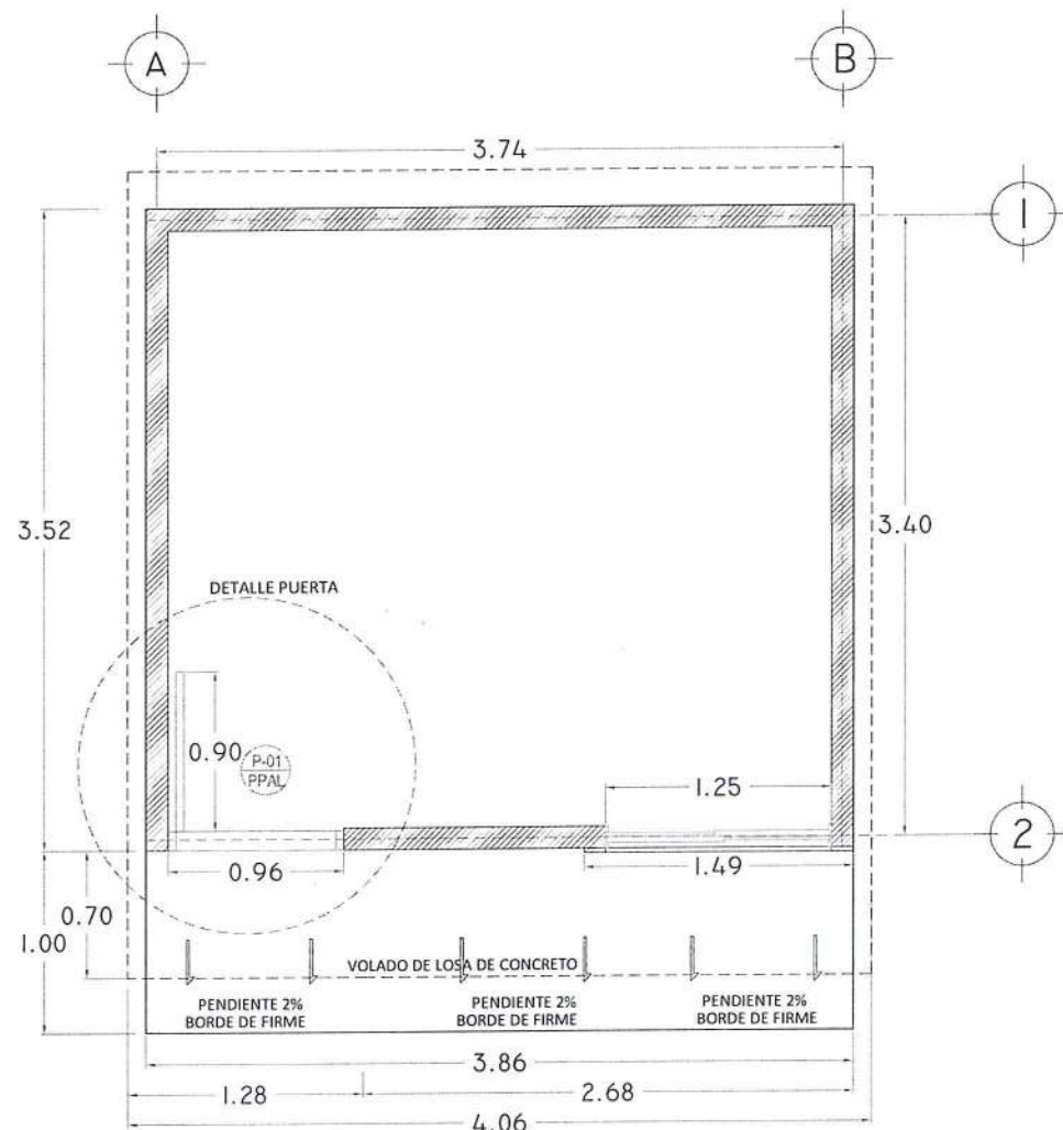
PLANTA ARQUITECTÓNICA
