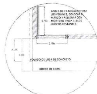
PLANTA DETALLE DE ANCLAJE DE PUERTA
