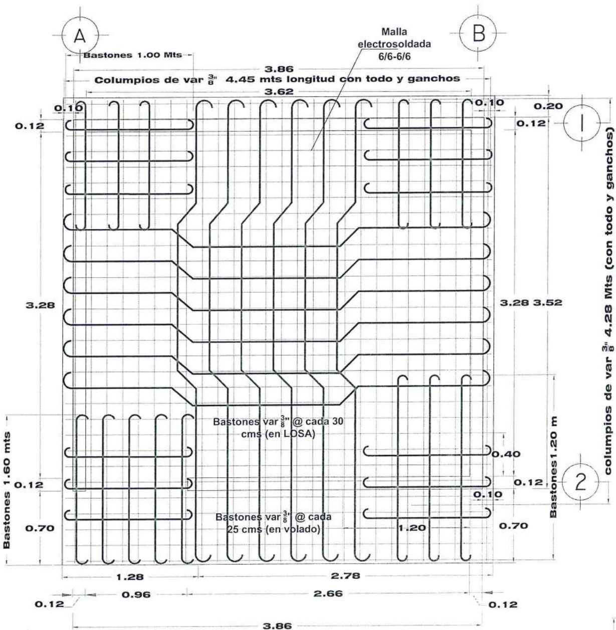
PLANTA DE ARMADO DE LOSA DE AZOTEA
