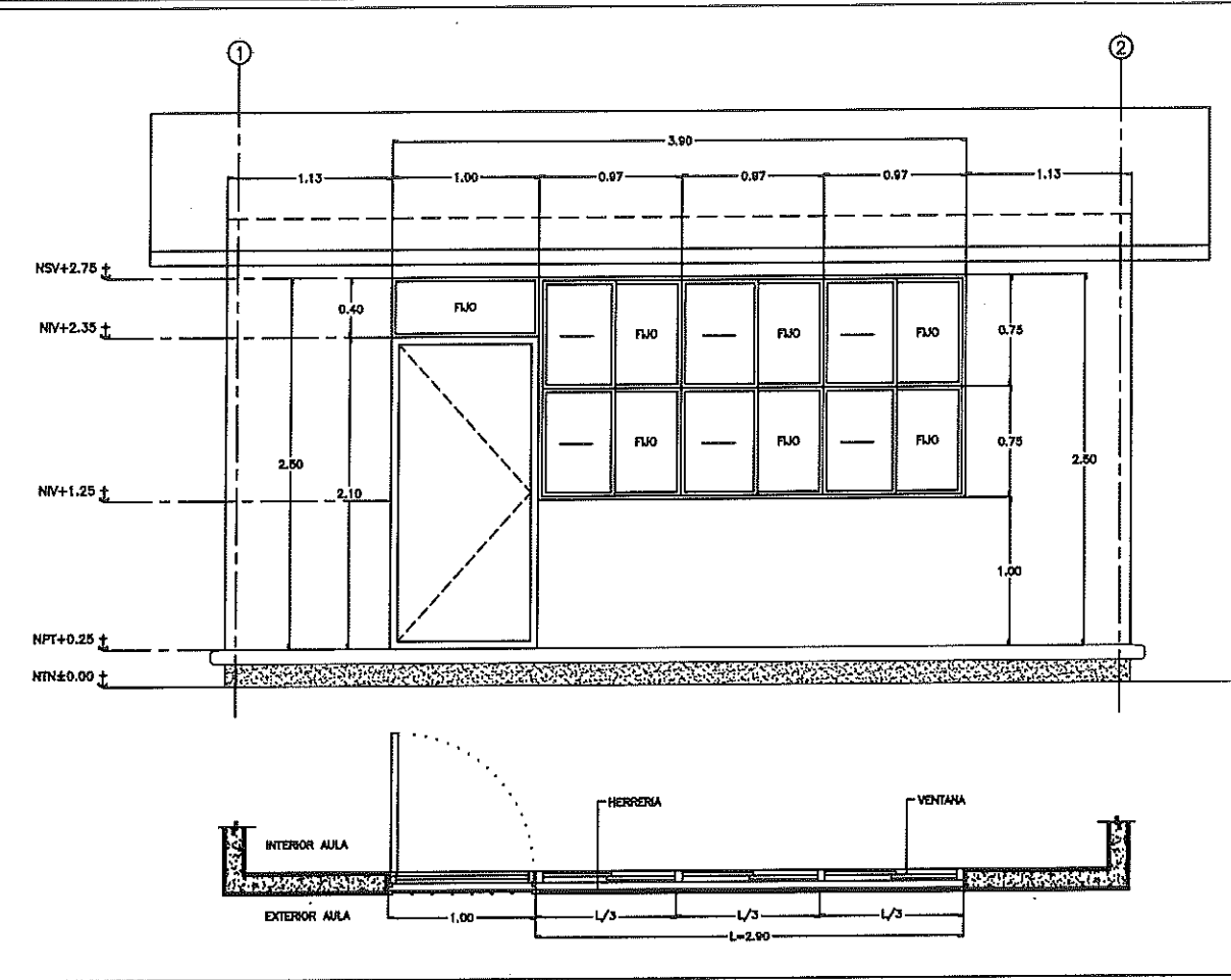
2 CANCELERIA EN FACHADA PRINCIPAL-AULAS ESC. 1:50
