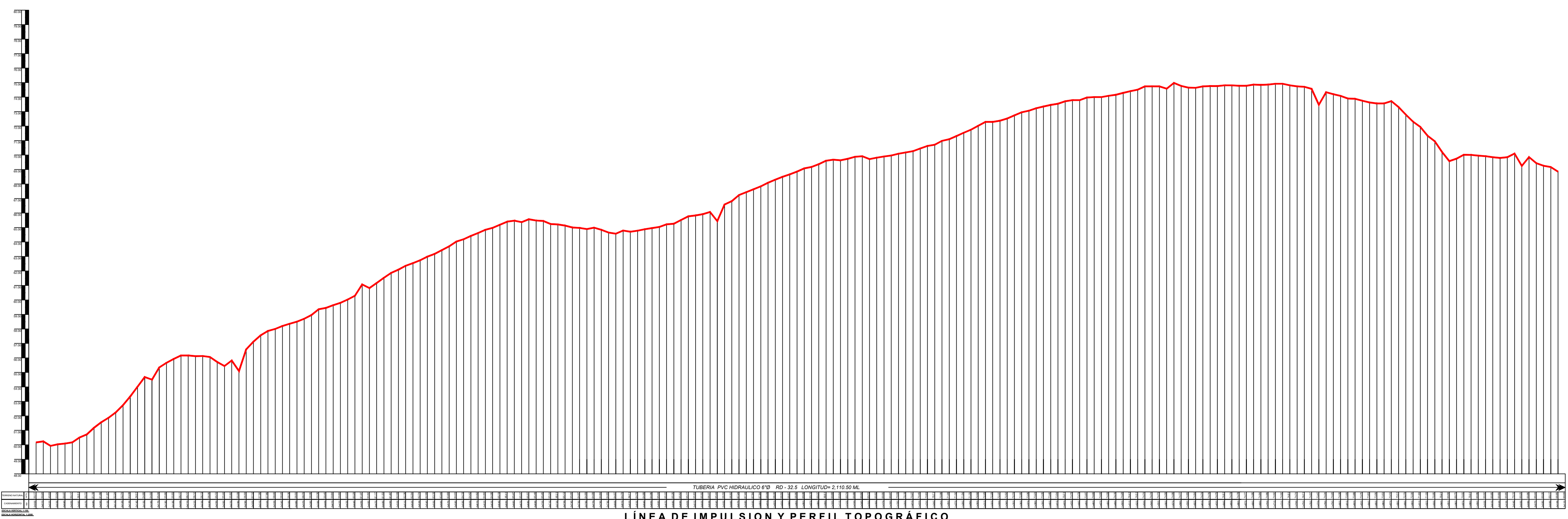
LÍNEA DE IMPULSION Y PERFIL TOPOGRÁFICO
