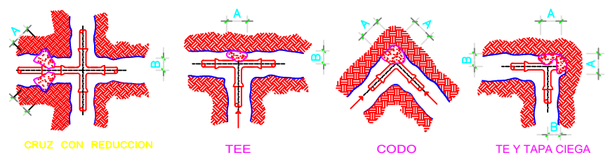
ATRAQUES PARA PIEZAS ESPECIALES SIN ESCALA
