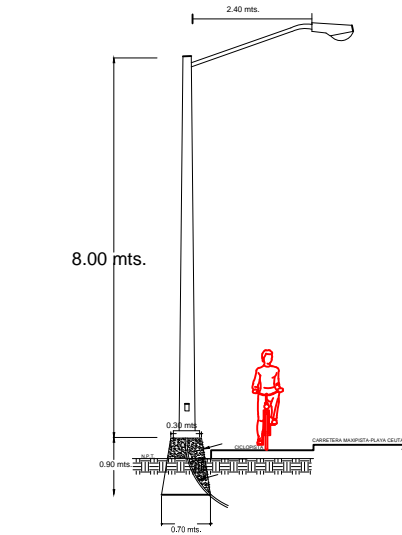
DETALLE EN ALZADO DE LUMINARIA
