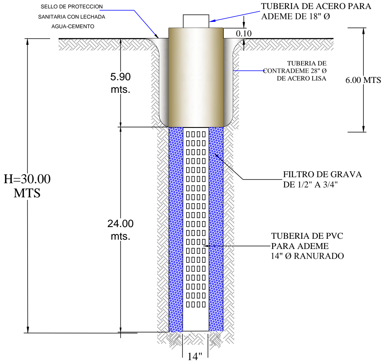
DETALLE DE POZO PROFUNDO
