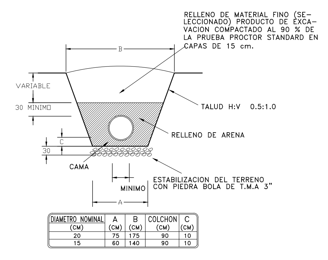
DETALLE DE ZANJA
