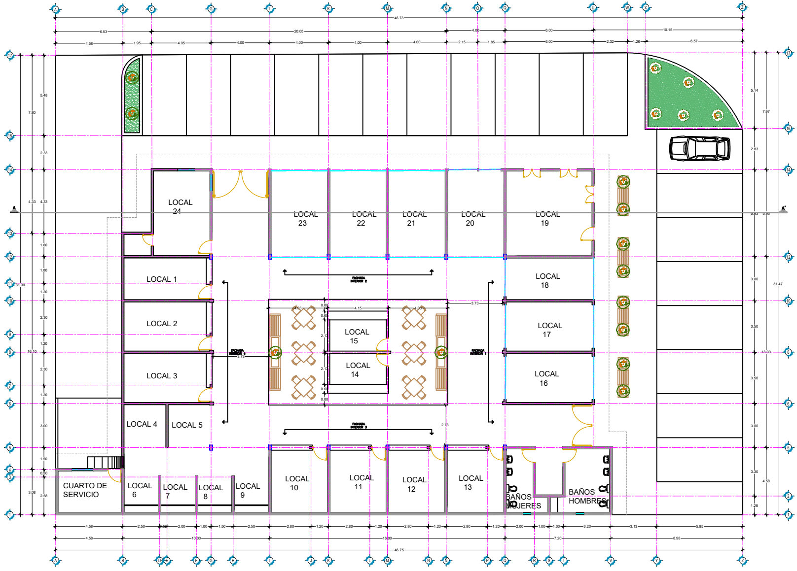
PLANTA ARQUITECTÓNICA
