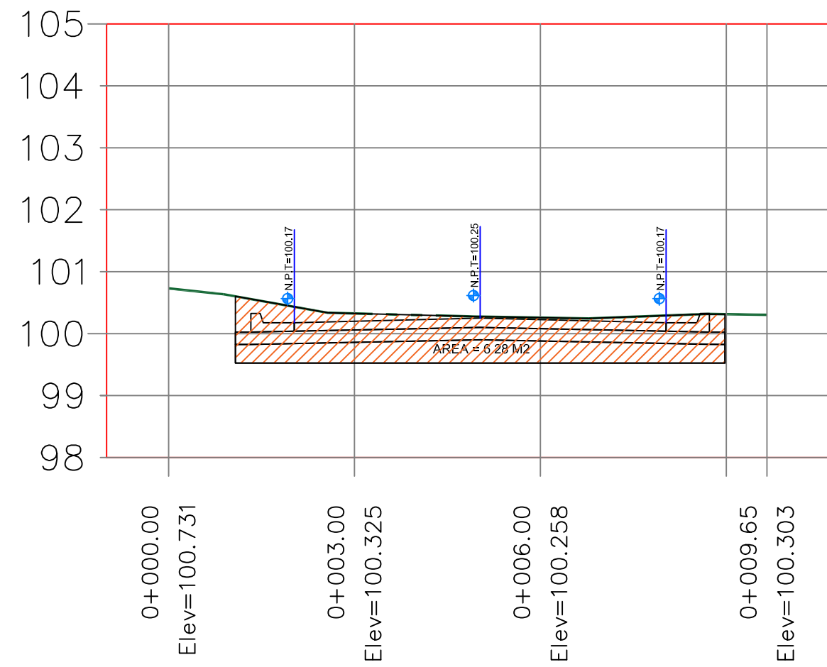
PERFIL 0+040
