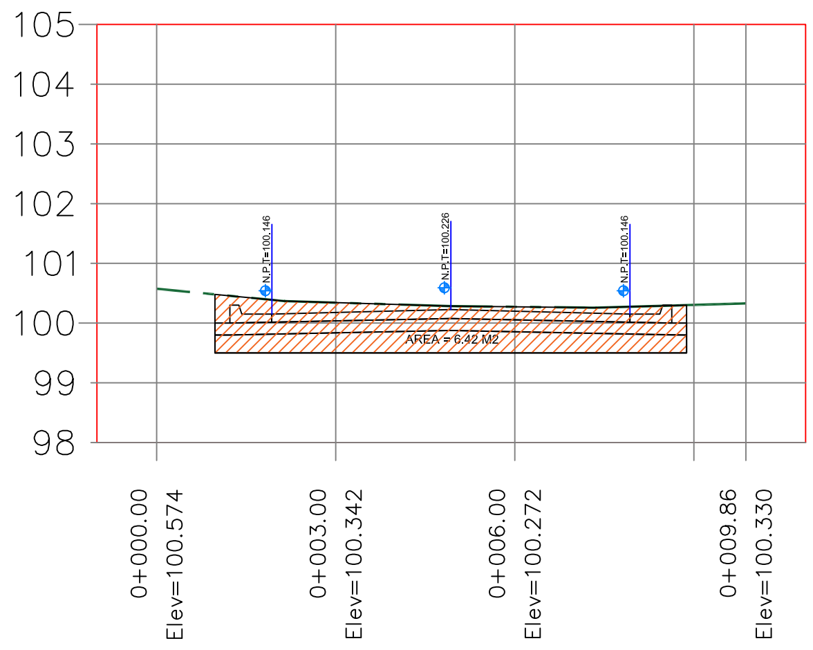
PERFIL 0+050
