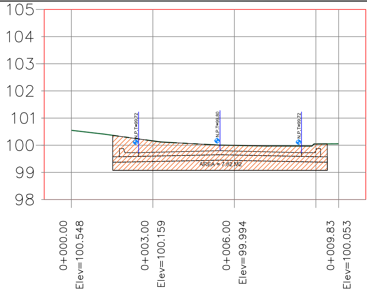
PERFIL 0+020
