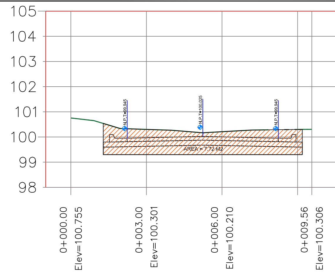
PERFIL 0+030
