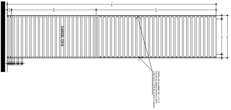
PS-01 (Alzado) PARASOLES PARA CANCEL C010
