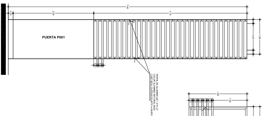
PS-02 (Alzado) PARASOLES PARA PUERTA P001
