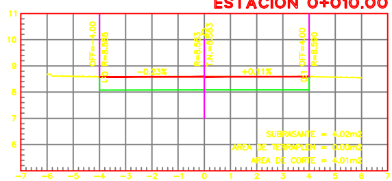
SECCIONES CALLE TERCERA (TRAMO 1)
