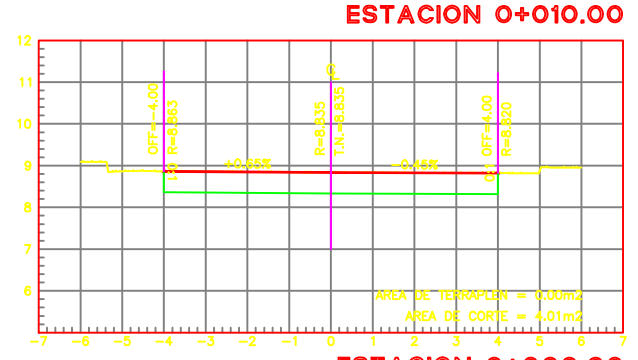
SECCIONES CALLE TERCERA (TRAMO 2)
