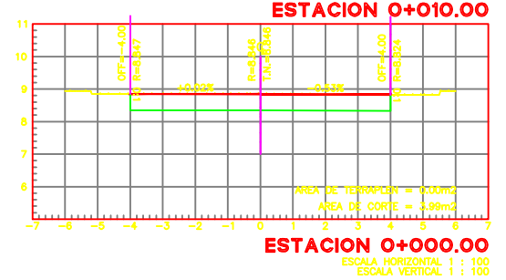
SECCIONES CALLE TERCERA (TRAMO 3)
