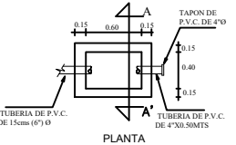
REGISTRO DE BANQUETA TIPO
