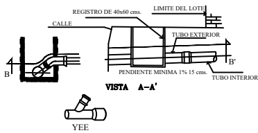
DESCARGA DOMICILIARIA CON TUBERIA DE P.V.C.
