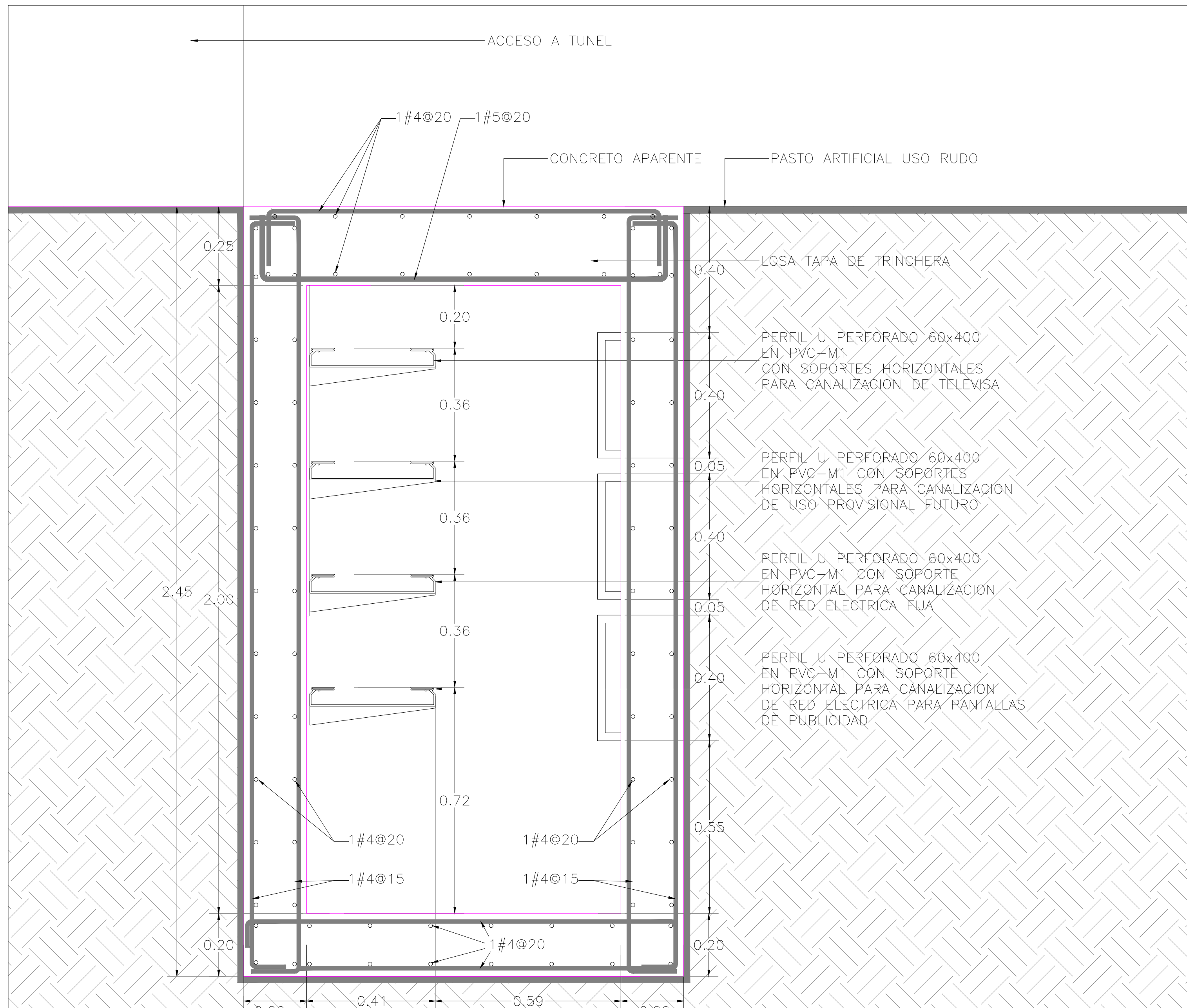
01 SECCION TRINCHERA 1:20 CANALIZACION DEBAJO DE TUNELES TR-244
