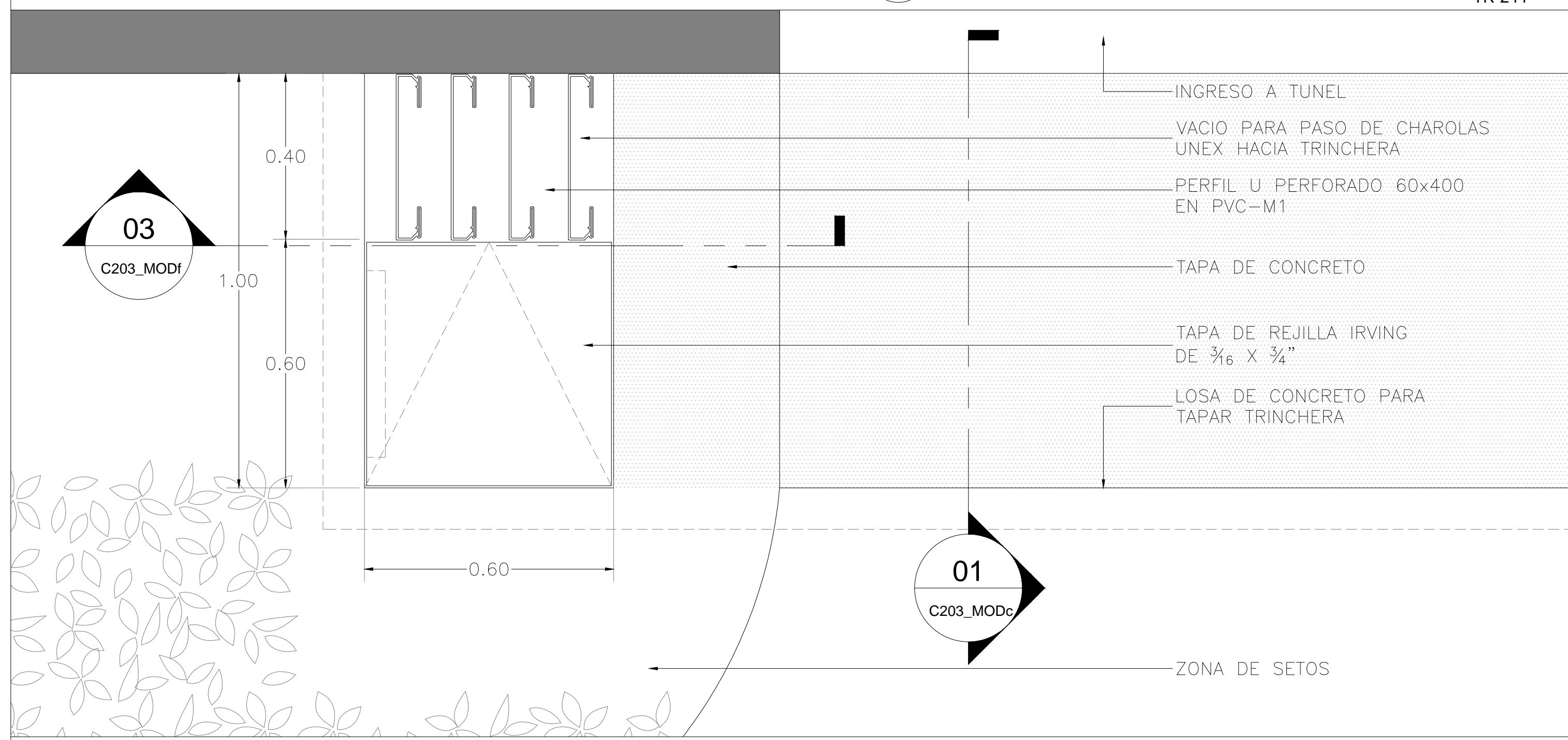
02 PLANTA TAPA DE TRINCHERA 1:20 TR-244
