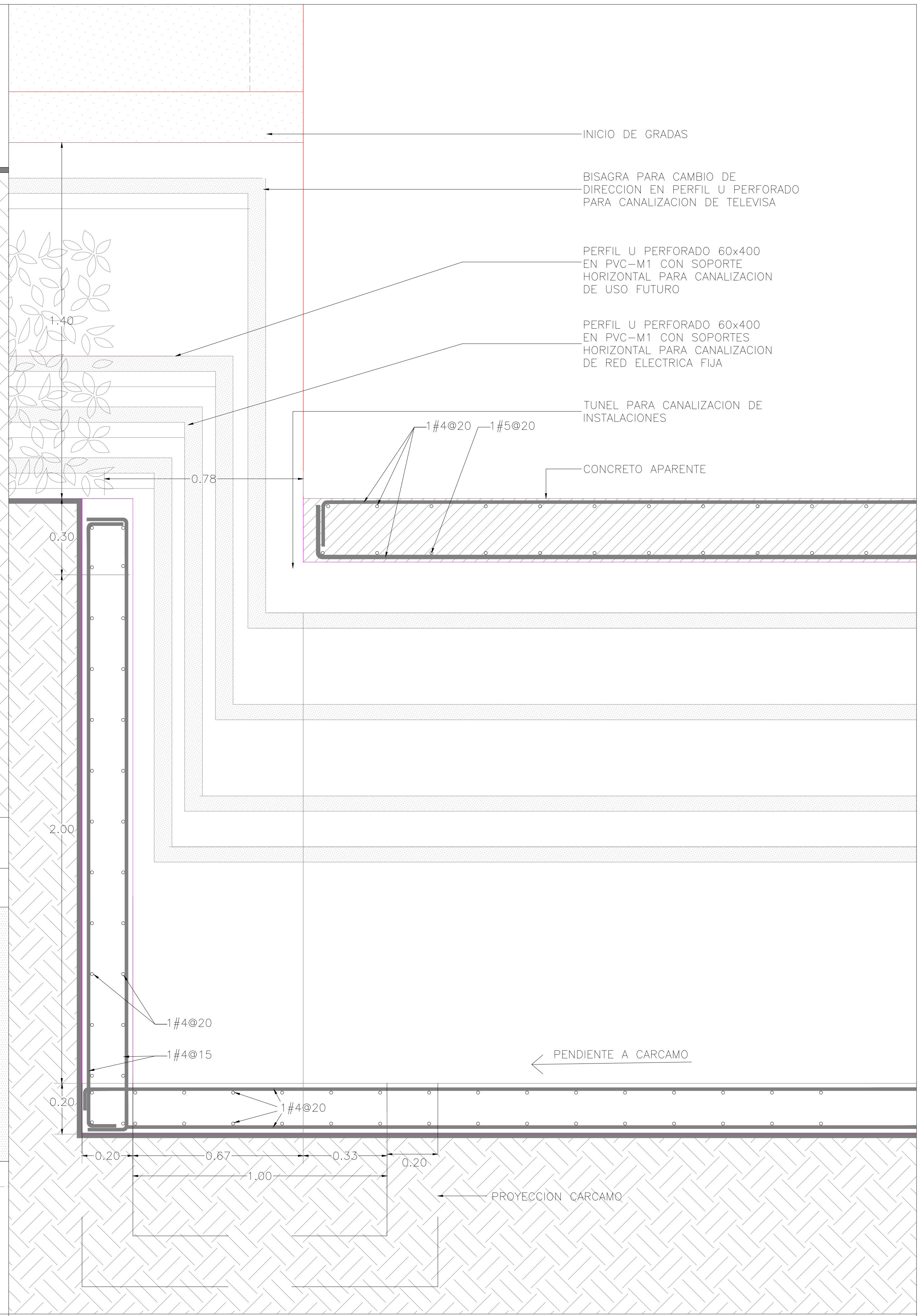
03 SECCION TRINCHERA 1:20 VISTA DEL CAMBIO DE DIRECCION EN CANALES TR-244
