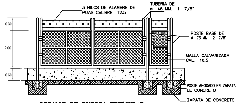
DETALLE DE PUERTA VEHICULAR SIN ESCALA
