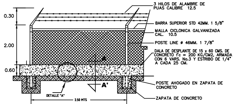
DETALLE DE MALLA CICLONICA SIN ESCALA
