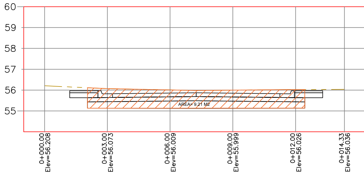
PERFIL 3
