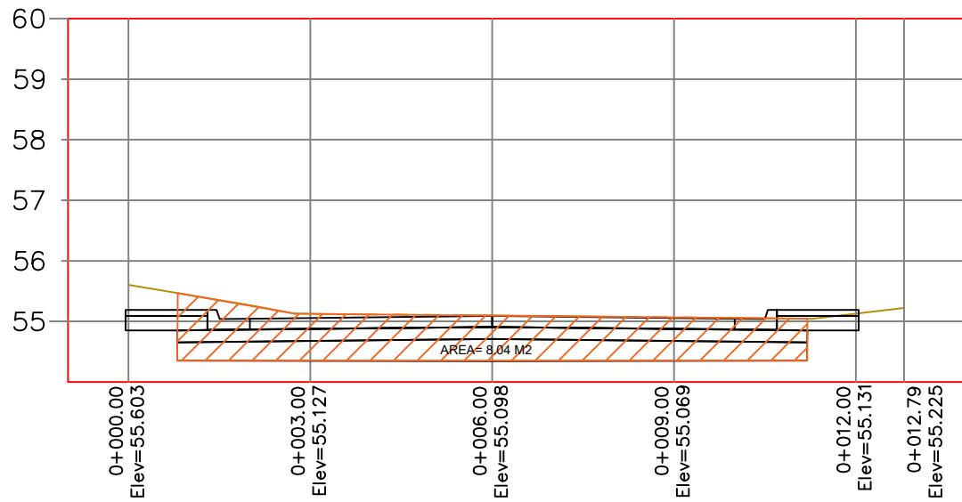
PERFIL 1
