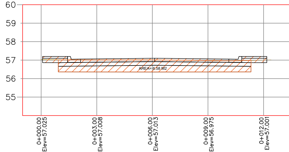
PERFIL 6
