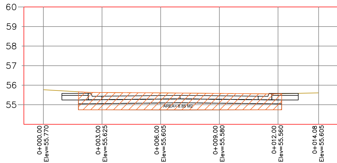
PERFIL 2
