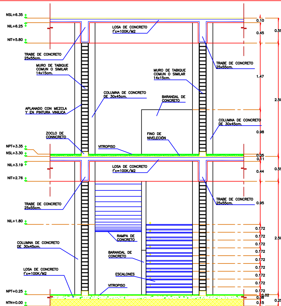
3 CORTE TRANSVERSAL
