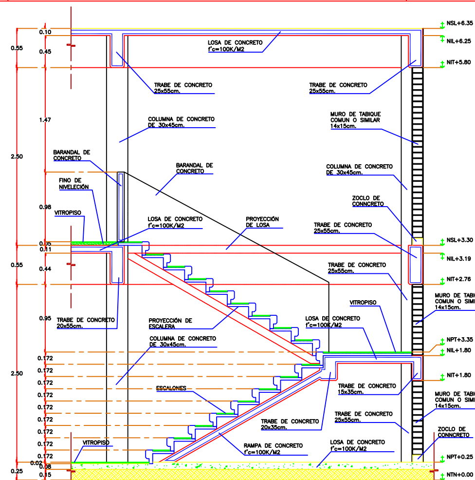
4 CORTE LONGITUDINAL
