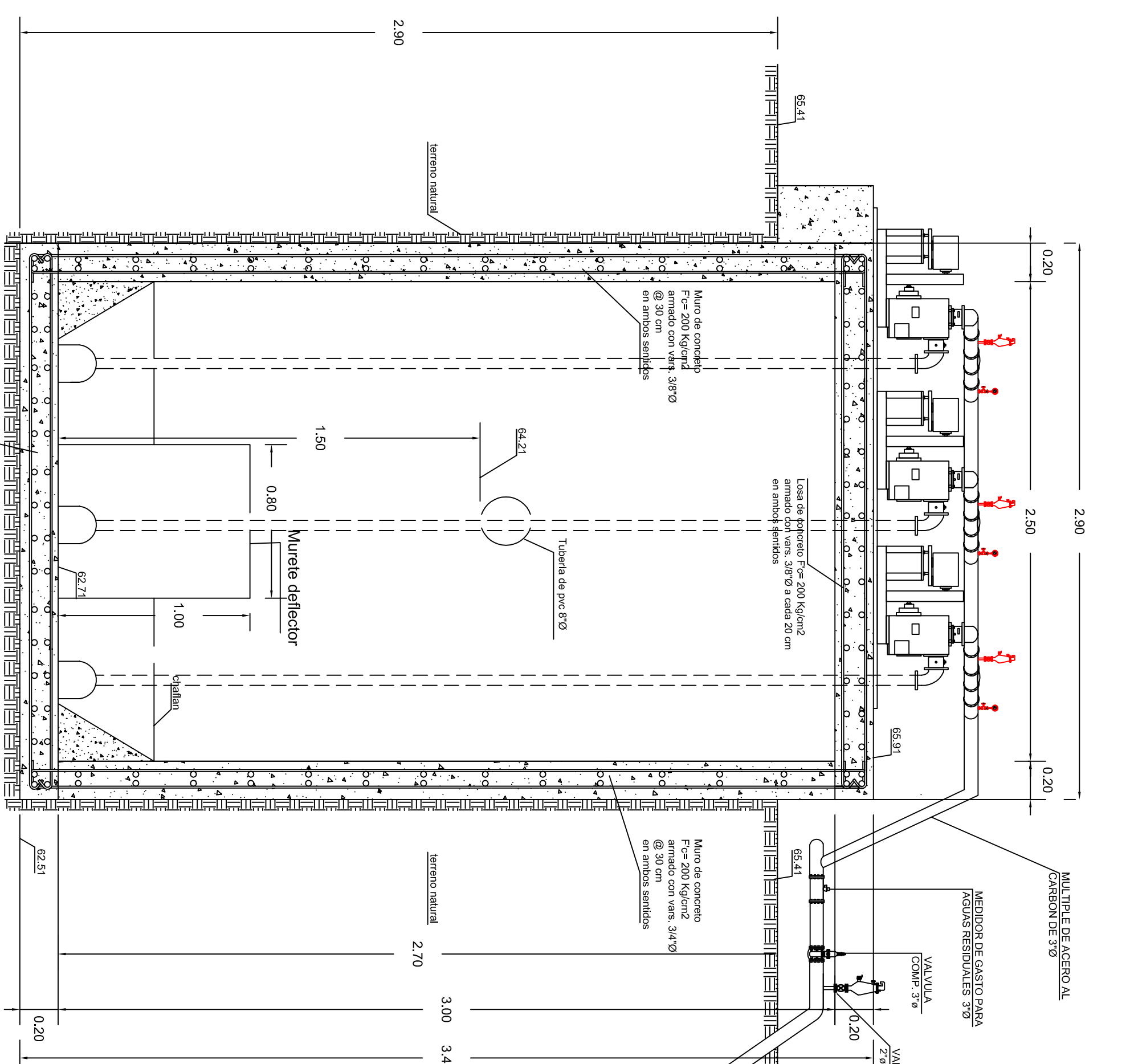
CORTE Y-Y
