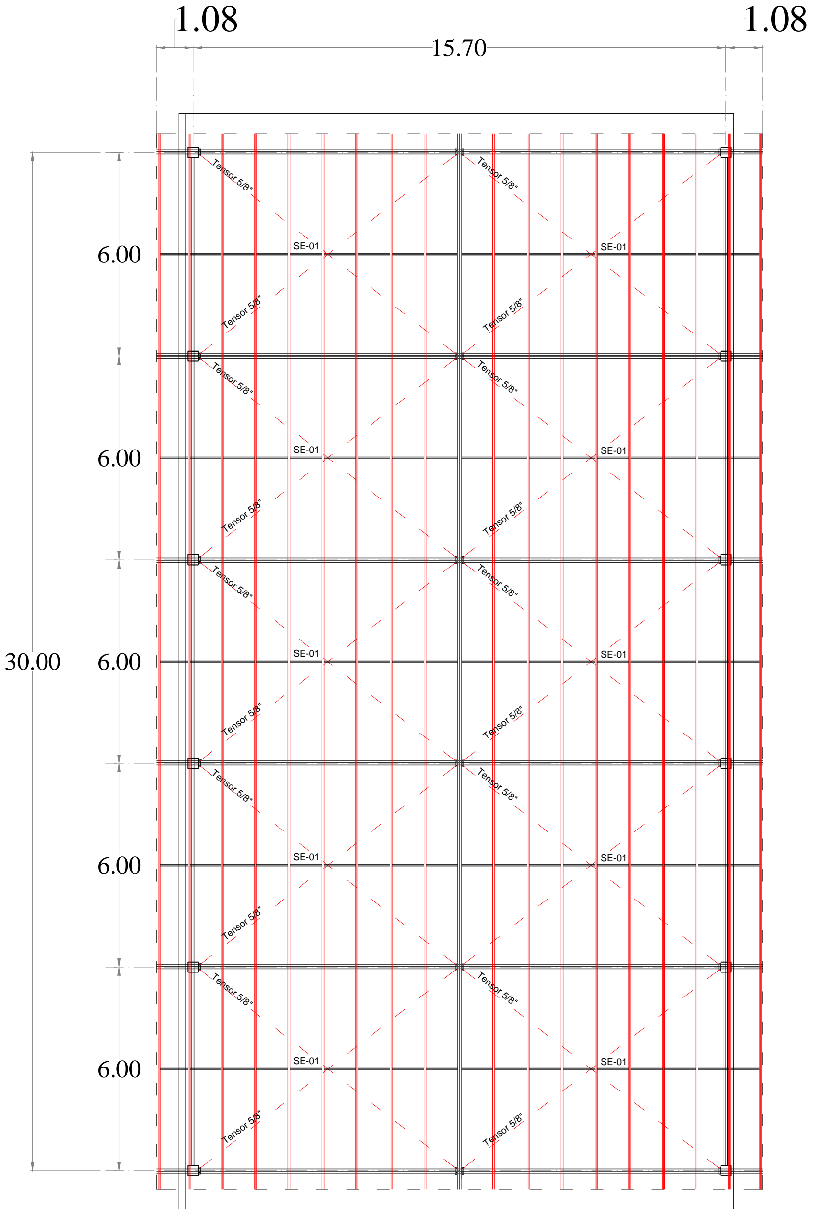
PLANTA ESTRUCTURAL DE CUBIERTA
