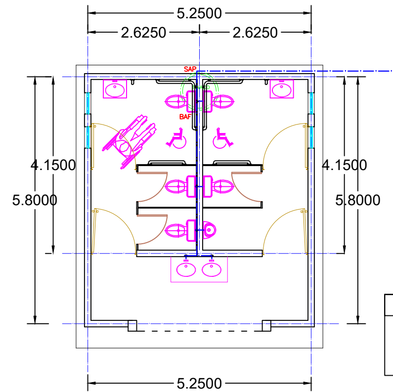
INSTALACION HIDRAULICA
