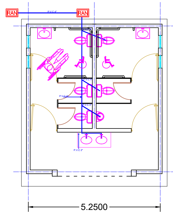
INSTALACION SANITARIA
