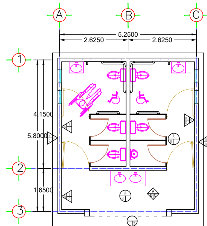
PLANTA DE ACABADOS
